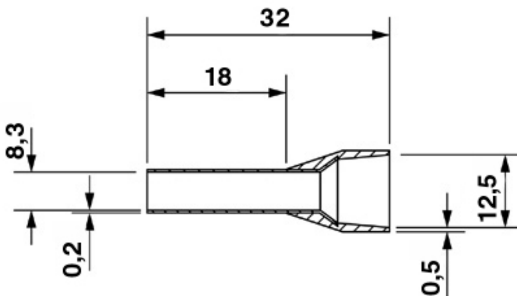
Чертеж
