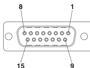
Схематический чертеж
