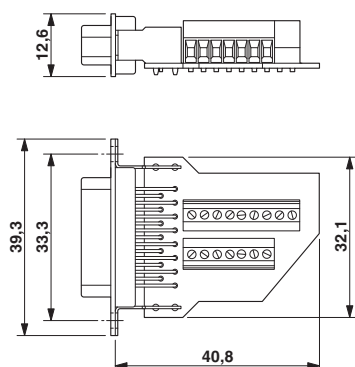
Чертеж
