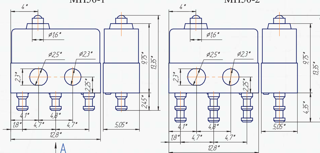
Габаритные и установочные размеры МП50-1 МП50-2
