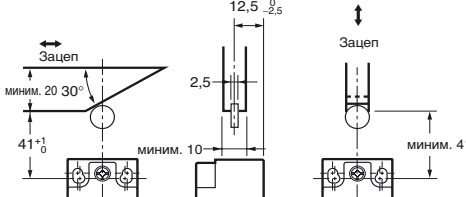
Однонаправленный рычаг с роликом (вертик.) (D4N-□□72R)
