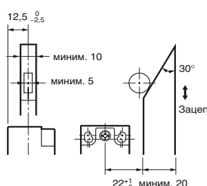
Однонаправленный рычаг с роликом (вертик.) (D4N-□□72R)
