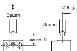
Герметизированный шток (D4N-□□31R)
