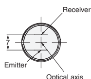
Suitable models E3FB-R□21 E3FB-D□2□ E3FB-L□2□
