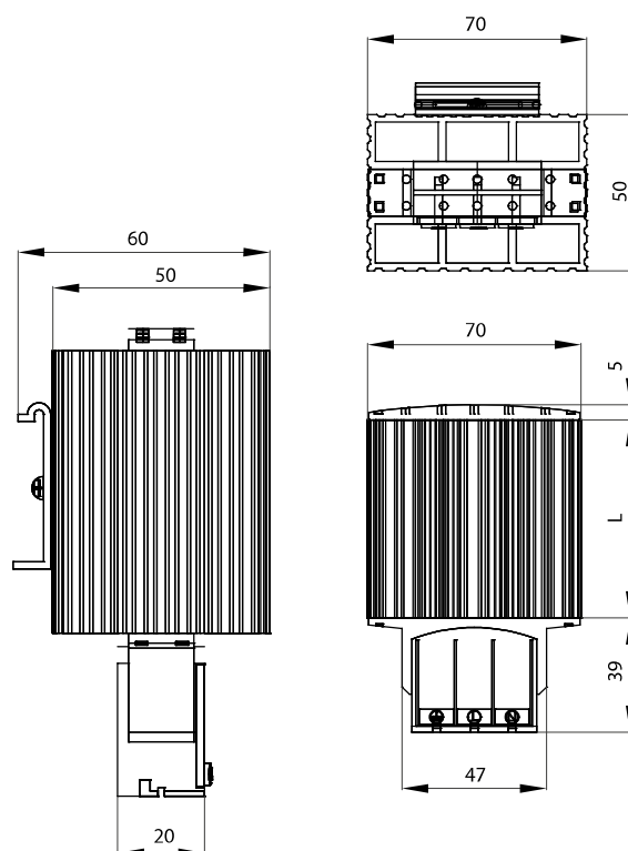
Габаритные и установочные размеры, мм
