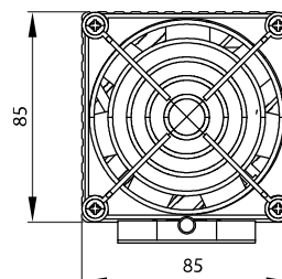
Габаритные и установочные размеры, мм
