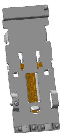
Комплект DIN-рейки для типоразмера А
