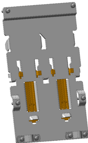
Комплект DIN-рейки для типоразмера В
