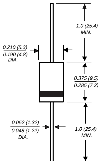
DO-201AD
