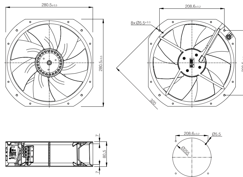
Габаритные и установочные размеры, мм
