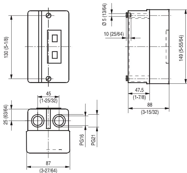
140-E41 (KT 3-25-KA)
