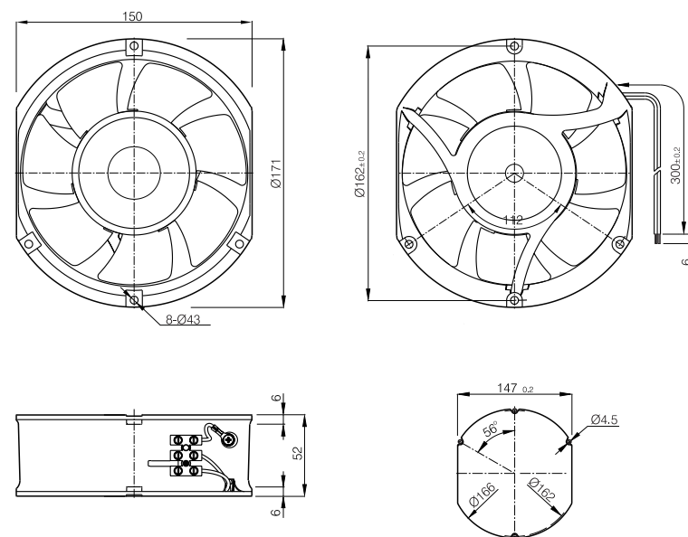
Габаритные и установочные размеры, мм
