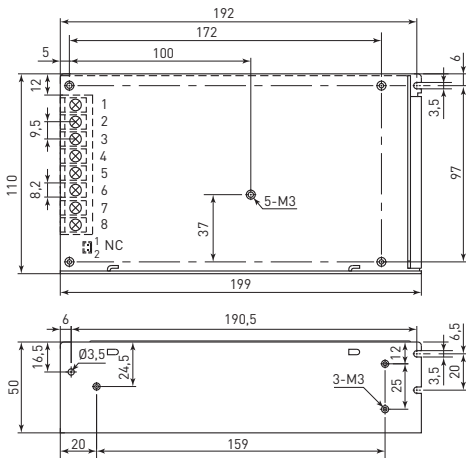
Рис. 2. Габаритные размеры MPSu-155W-24
