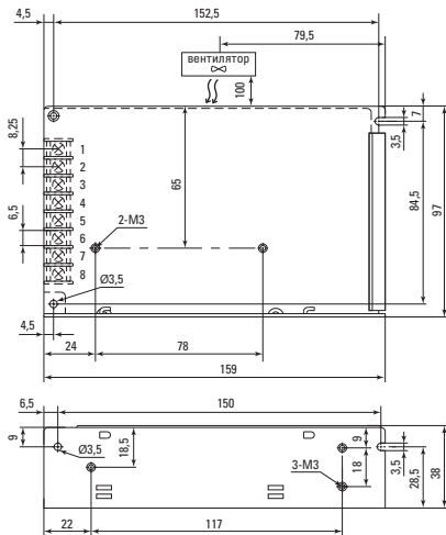
Рис. 1. Габаритные размеры MPSu-55W-24
