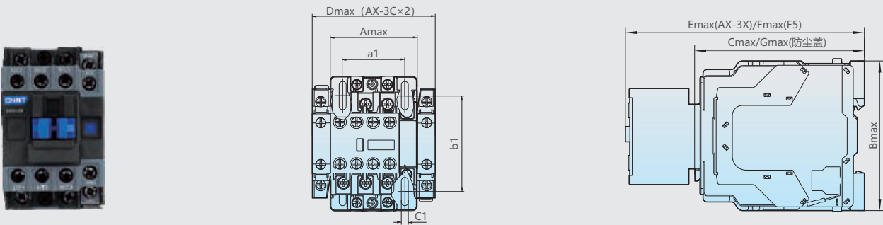
NXC-40~100 外形尺寸与安装尺寸
