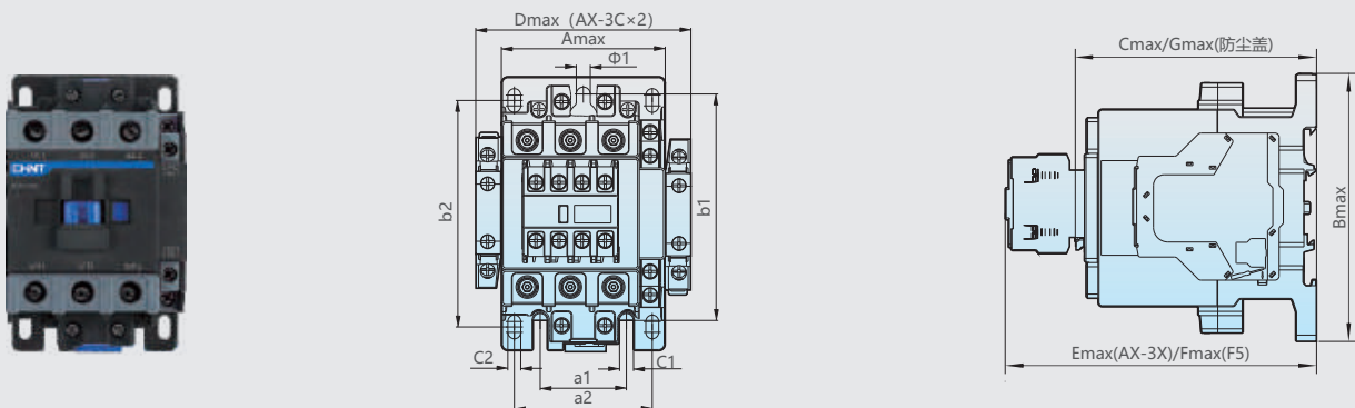
NXC-40~100 外形尺寸与安装尺寸
