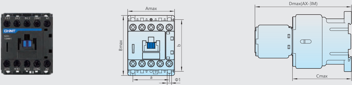
NXC-06M~12M 外形尺寸与安装尺寸
