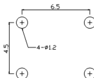
Монтажные отверстия на печатной плате
