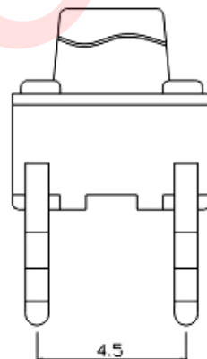
Монтажные отверстия на печатной плате
