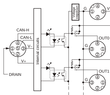
DRT2-OD08CL-1 (PNP)
