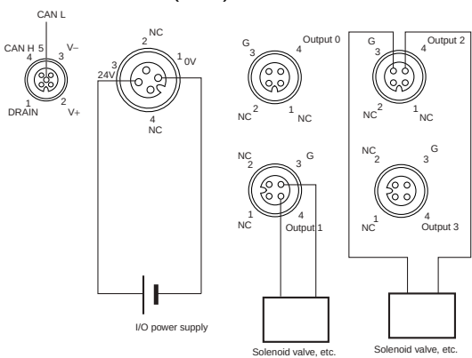
DRT2-OD04CL-1 (PNP)
