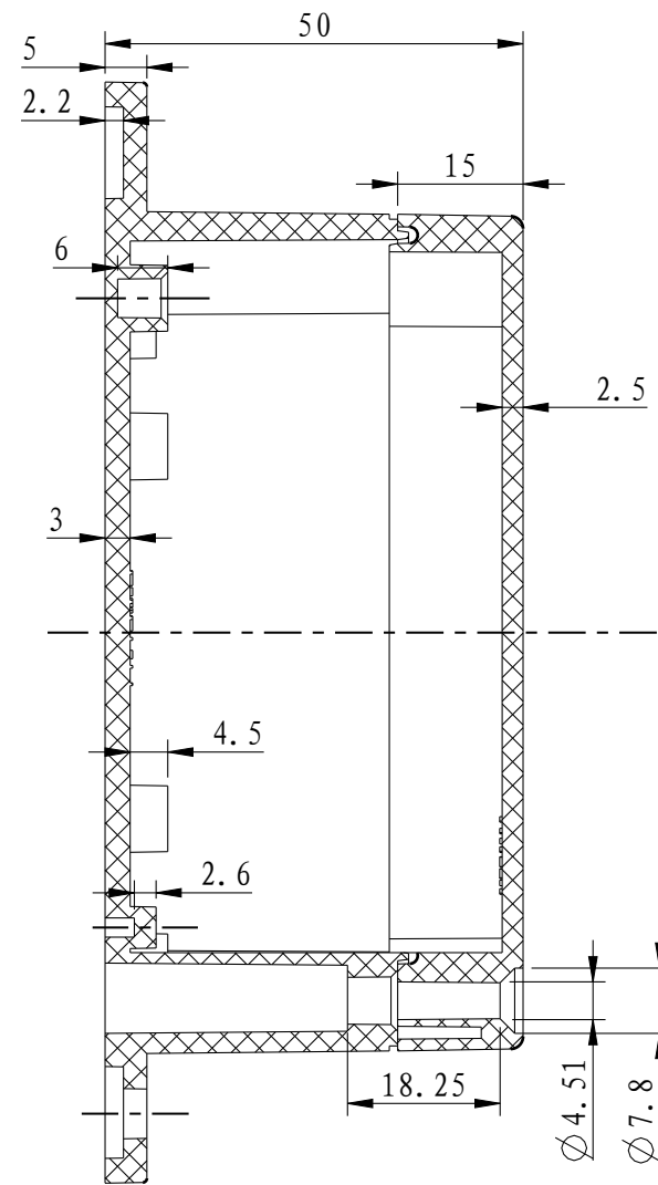
剖面 C-C
