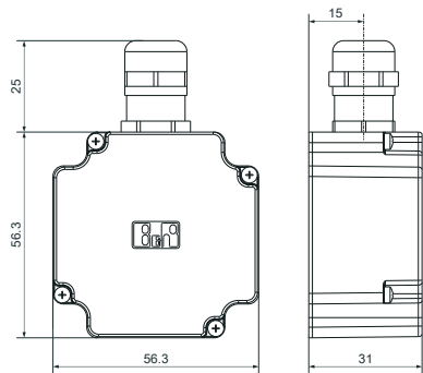
Размеры уплотняющей крышки для шаговых двигателей 80MPD и 80MPF (все размеры в мм)
