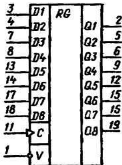
Условное графическое обозначение К556ИР27
