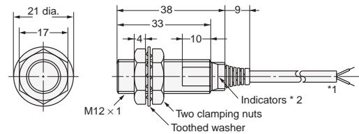
Diagram 5 E2E-X3D□ E2E-X2E□/F□
