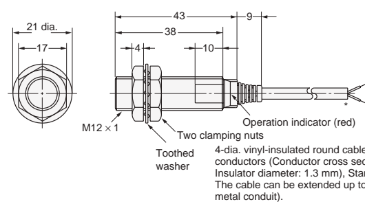
Diagram 7 E2E-X2Y□
