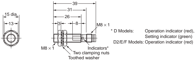
Diagram 24 E2E-X2D□-M3G/E2E-X1R5E□-M3/X1RF□-M3
