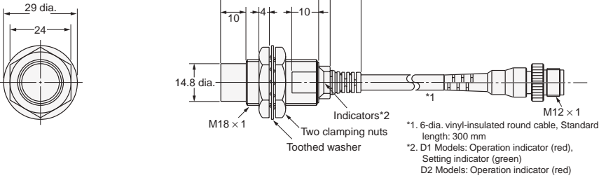
Diagram 32 E2E-X14MD□-M1GJ E2E-X14MD1-M1TGJ E2E-X14MD□-M1TGJ-US
