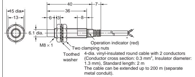
Diagram 6 E2E-X8MD□ E2E-X5ME□/F□
