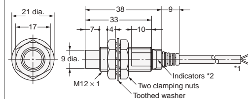
Diagram 6 E2E-X8MD□ E2E-X5ME□/F□
