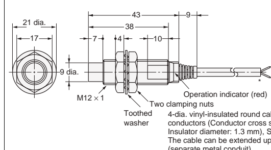
Diagram 8 E2E-X5MY□
