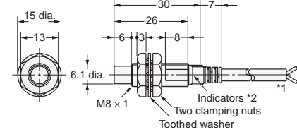
Diagram 2 E2E-X4MD□ E2E-X2ME□/F□
