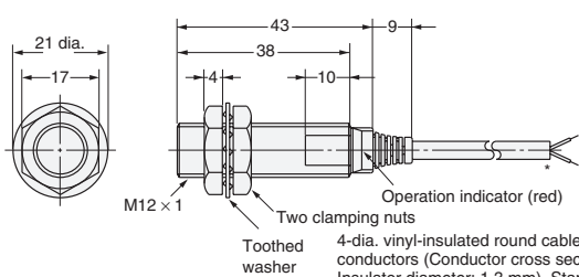
Diagram 7 E2E-X2Y□
