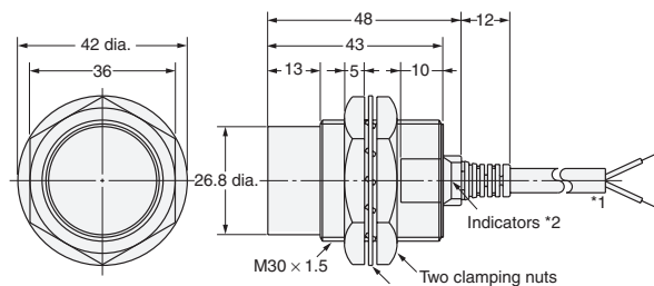
Diagram 13 E2E-X20MD□/E2E-X18ME□/F□ E2E-X18MY□
