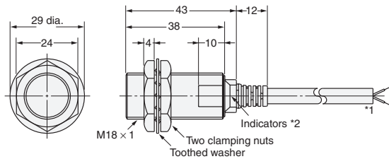
Diagram 10 E2E-X7D□/E2E-X5E□/F□ E2E-X5Y□/E2E-X7T1
