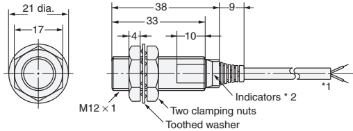
Diagram 5 E2E-X3D□ E2E-X2E□/F□
