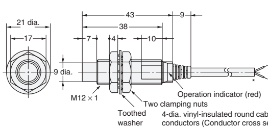
Diagram 8 E2E-X5MY□
