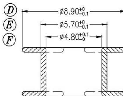
SEC A-A
