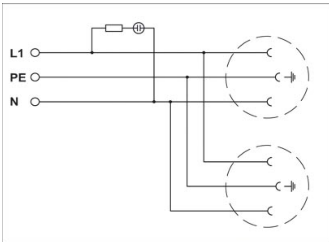
Электрическая схема
