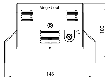
Габаритные и установочные размеры, мм
