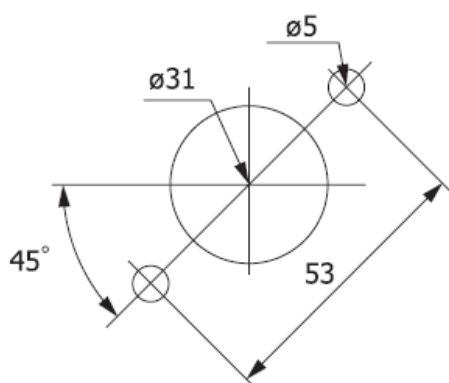
Рис.25 – Размеры выреза для ручки
