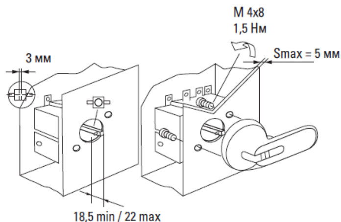
Рис. 24 – Установка рукоятки для управления через дверь
