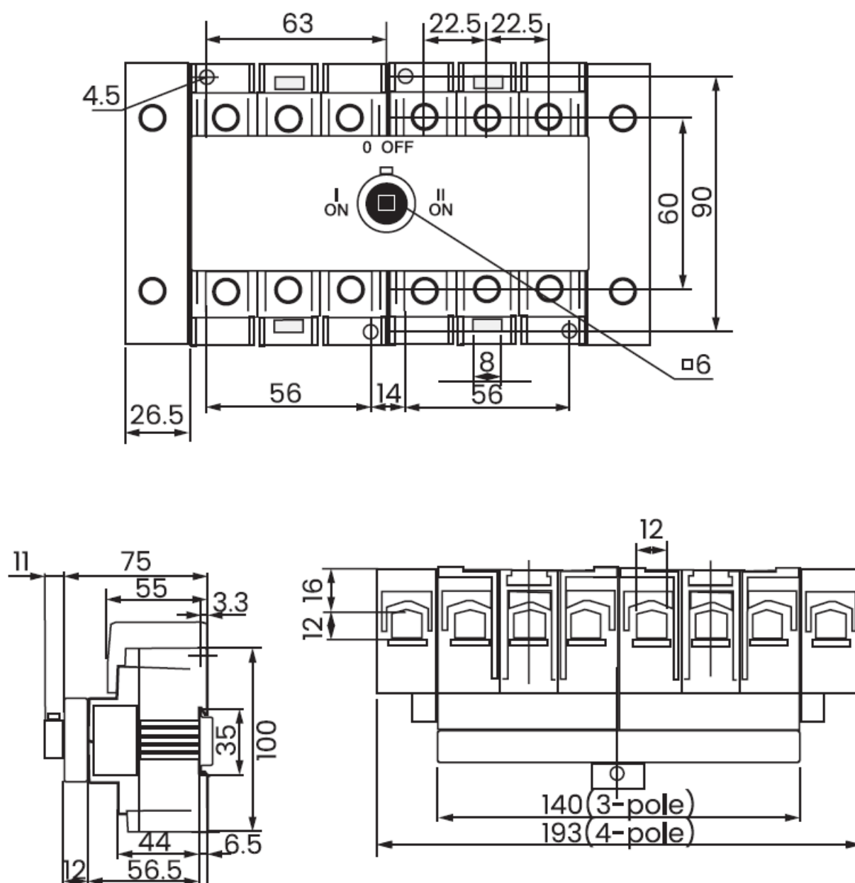
Рис. 12 – Габаритные и установочные размеры реверсивных рубильников 40-125А 3Р-4Р
