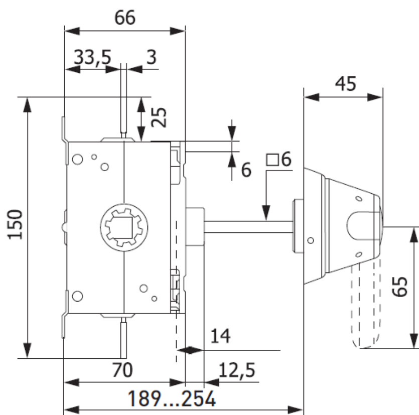
Рис. 3 – Габаритные и установочные размеры рубильников 160-250 А 3Р
