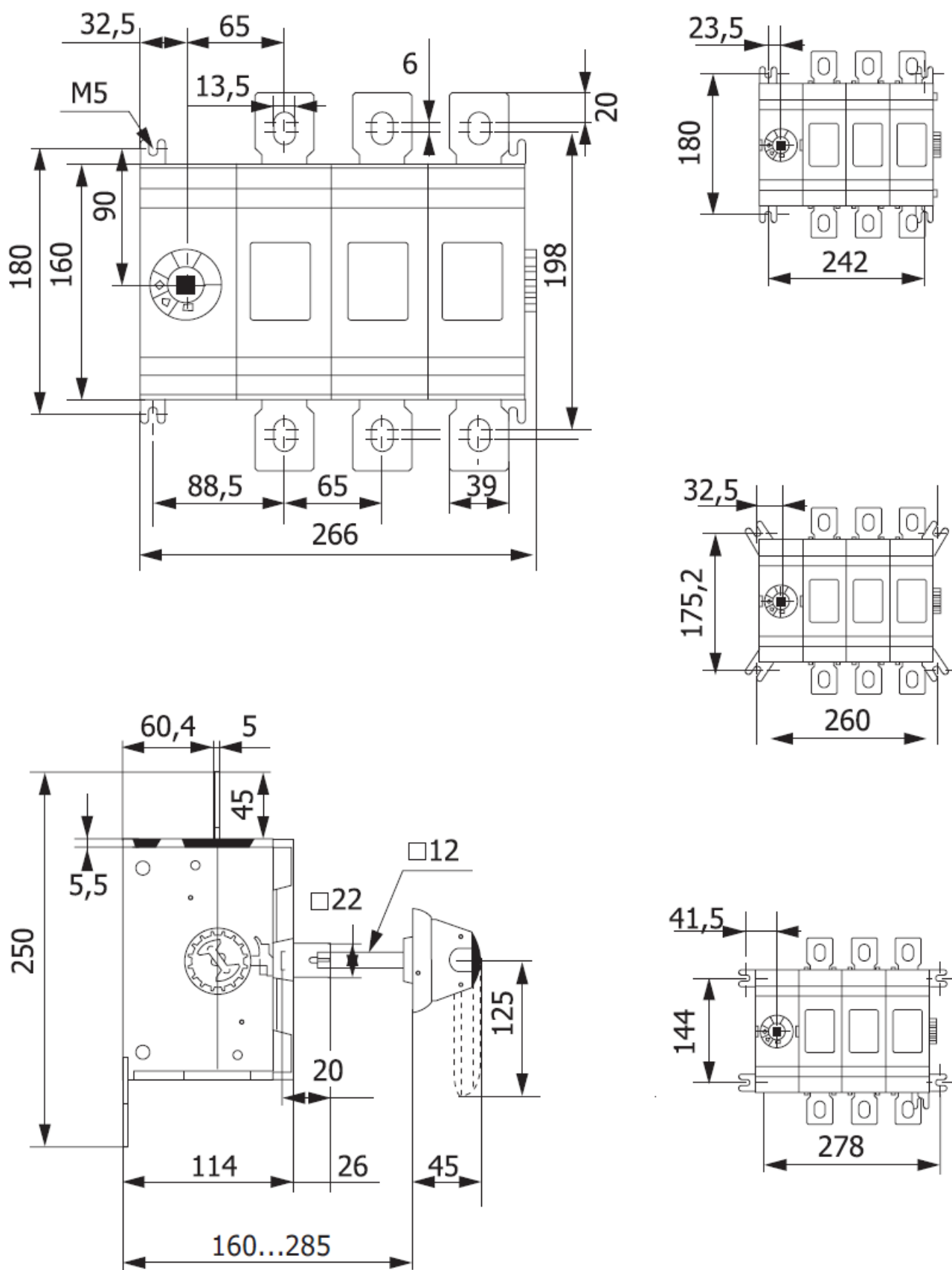
Рис. 7 – Габаритные и установочные размеры рубильников 630-800 А 3Р
