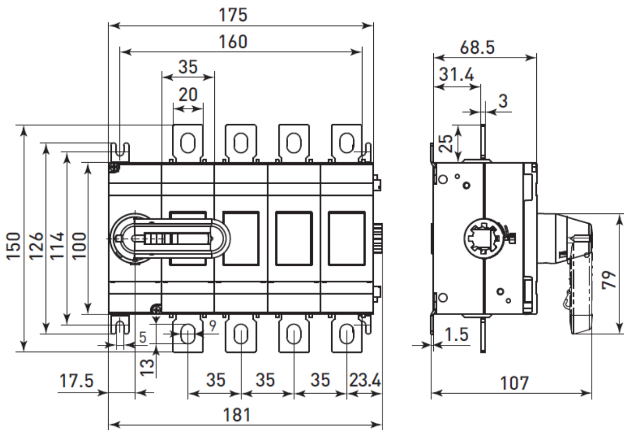
Рис. 5 – Габаритные и установочные размеры рубильников 160-250 А 4Р
