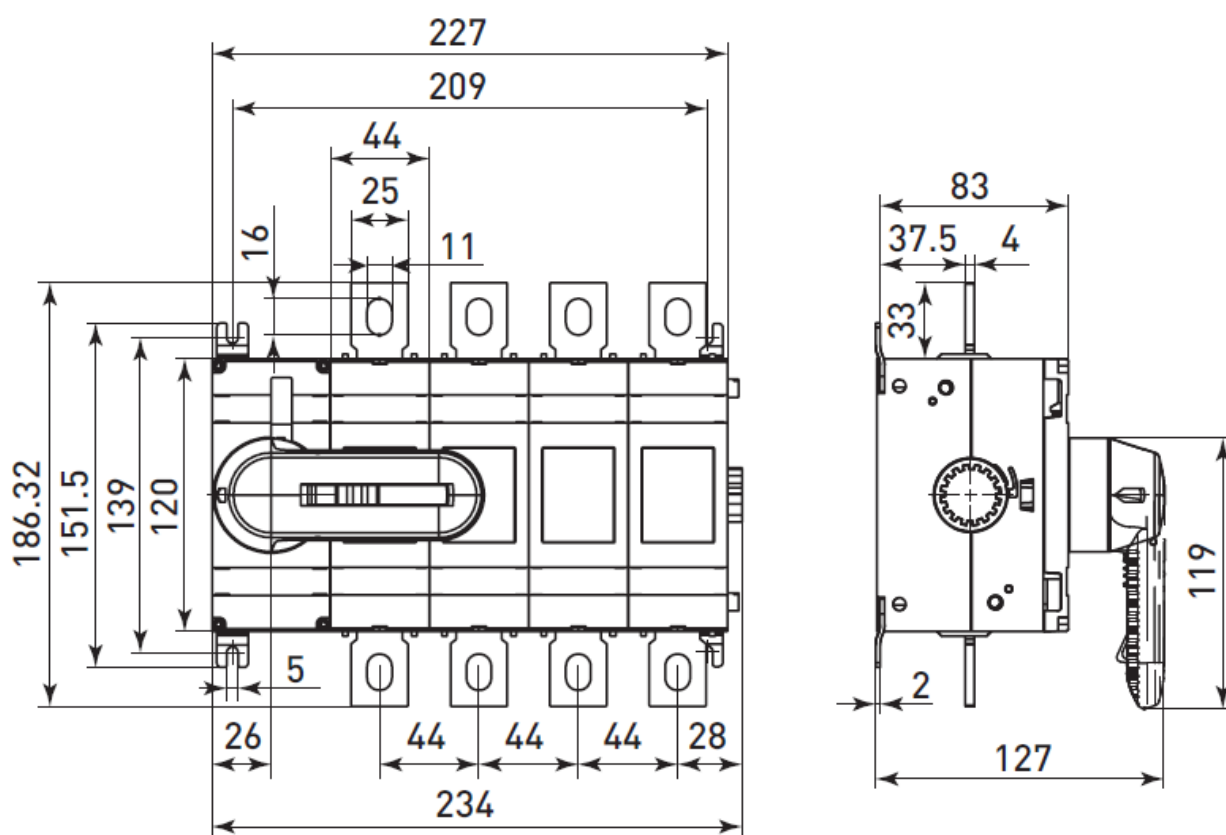
Рис. 6 – Габаритные и установочные размеры рубильников 315-400 А 4Р
