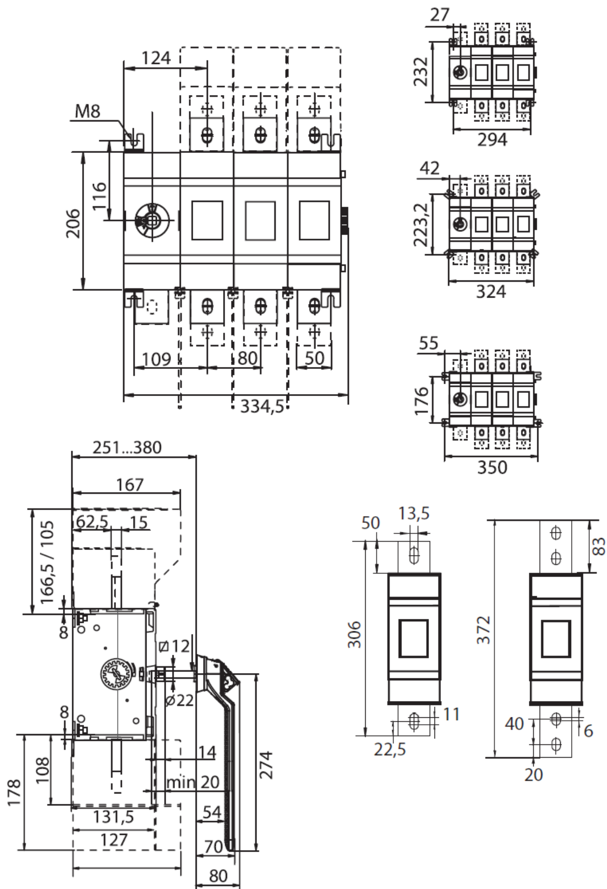
Рис. 8 – Габаритные и установочные размеры рубильников 1000-1600 А 3Р
