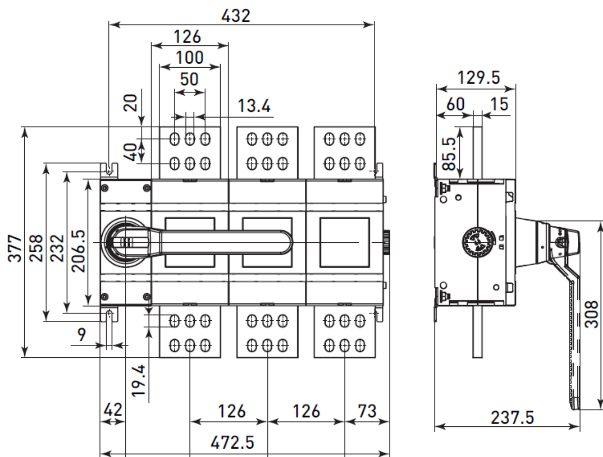
Рис. 11 – Габаритные и установочные размеры рубильников 2000-2500 А 3Р
