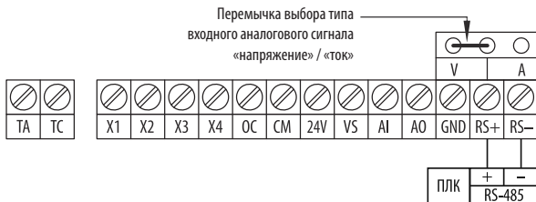
Рисунок 26 – схема подключения ПЧ к ПЛК по интерфейсу RS-485.
