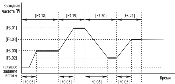
Рисунок 54 – режим программы ПЛК «Один цикл и работа на последней (четвертой) скорости».
