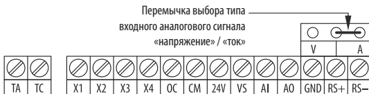
Рисунок 10 – Клеммы цепей управления.
