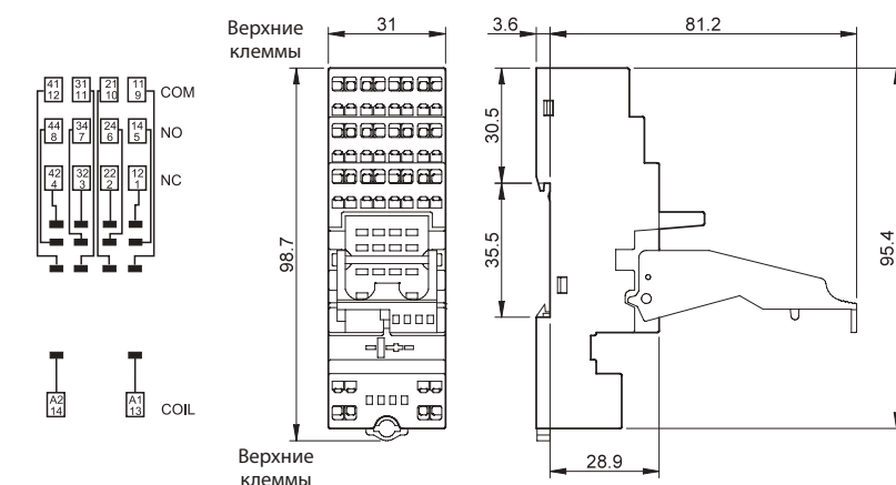
Розетка + 6-полюсная перемычка
