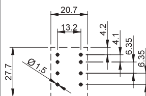
Вид со стороны выводов
