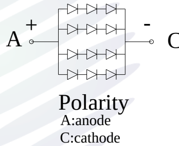
Fig.1-4 Polarity 极性
