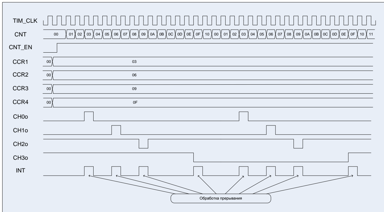
Рисунок 92 – Диаграммы примера работы в режиме ШИМ
