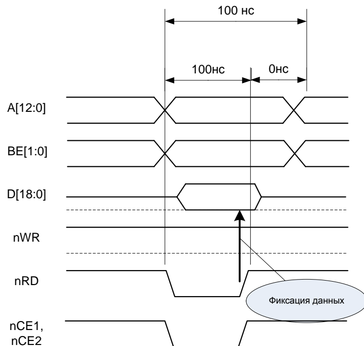
Рисунок 35 – Временная диаграмма цикла чтения
