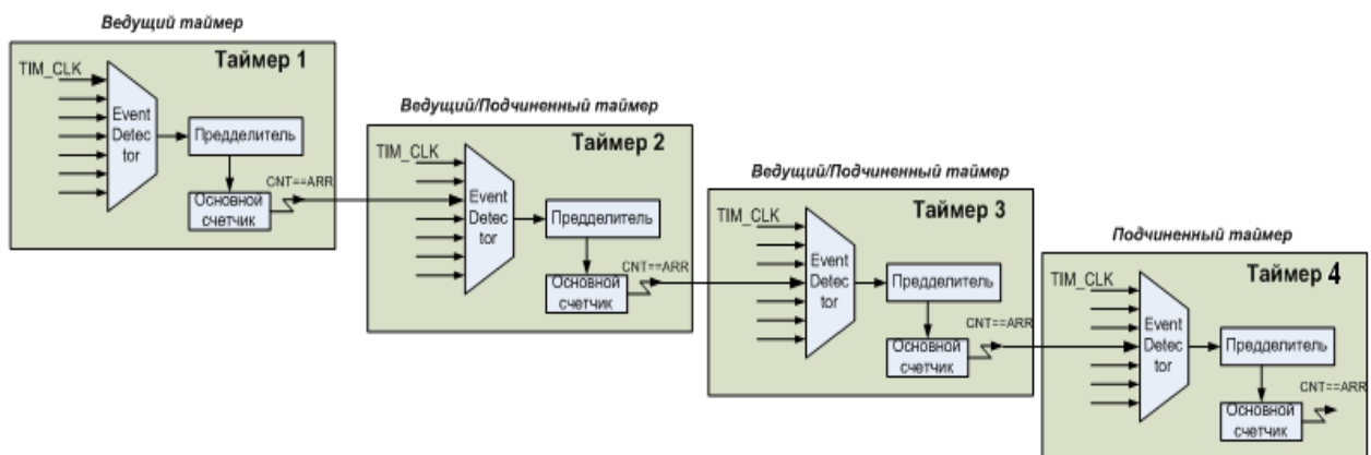
Рисунок 74 – Пример каскадного соединения таймеров
