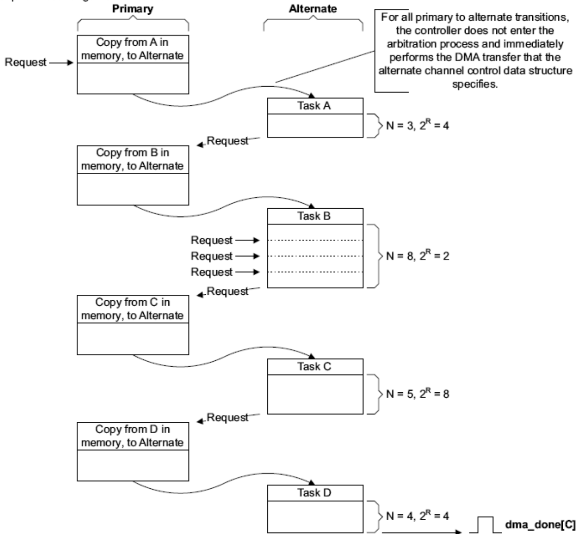
Рисунок 133 – Пример работы DMA в режиме с «Исполнением с изменением конфигурации»
