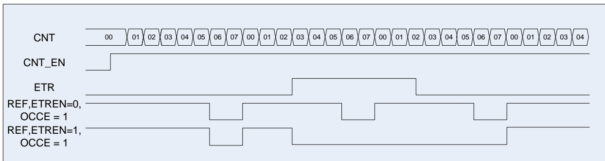
Рисунок 87 – Диаграмма работы схемы в режиме ШИМ, CCR1_EN = 0
