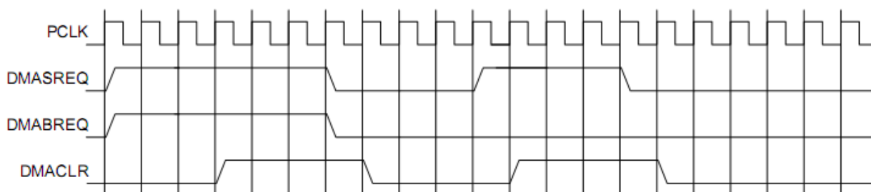
Рисунок 123 – Временные диаграммы одноэлементного и блочного запросов DMA
