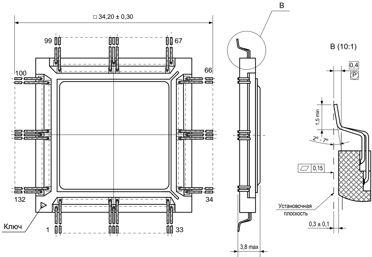
Рисунок 147 – Корпус 4229.132-3 с формованными выводами
