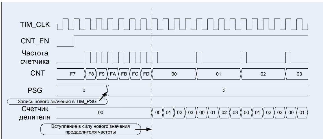
Рисунок 71 – Диаграммы работы счетчика: счет вверх (CNT_MODE = 00, EVENT_SEL = 0000, DIR = 0)
