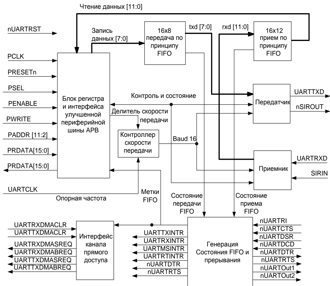
Рисунок 117 – Блок-схема универсального асинхронного приёмопередатчика (UART)
