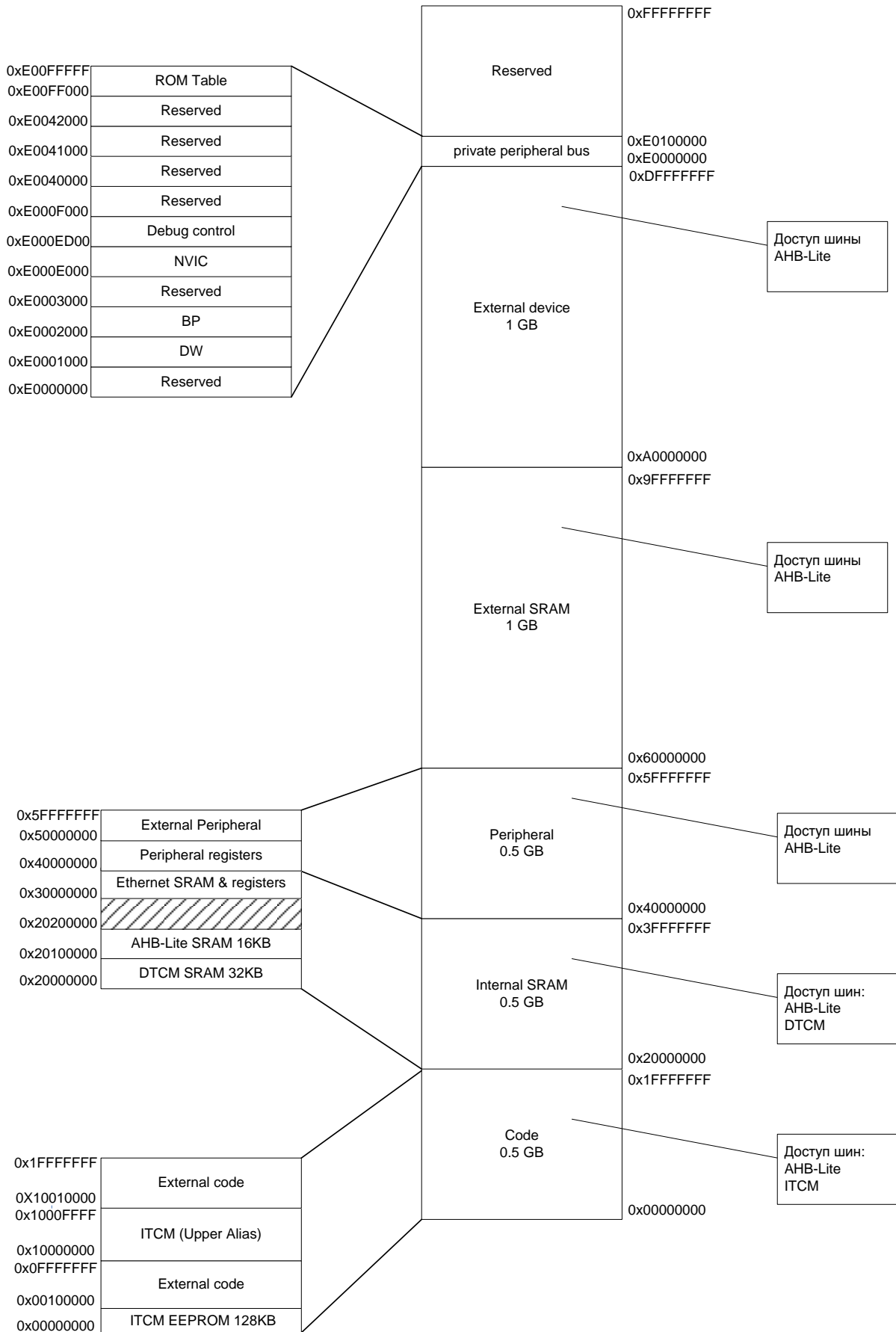
Рисунок 11 – Карта распределения основных областей памяти
