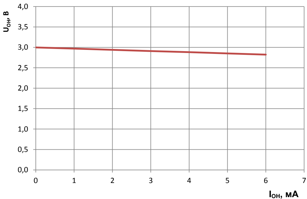
Рисунок 144 – Зависимость выходного напряжения высокого уровня от выходного тока высокого уровня при напряжении питания 3,0 В
