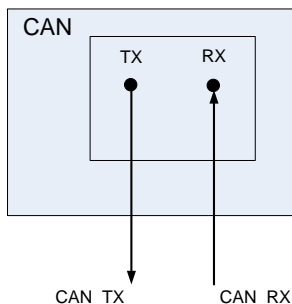
Рисунок 41 – Режим нормальной передачи
