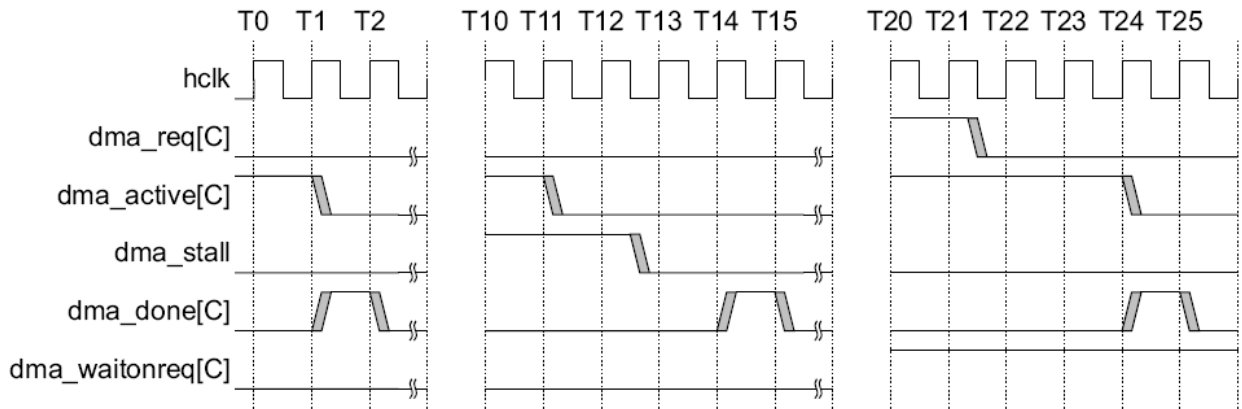
Рисунок 127 – Диаграммы функционирования dma_done
