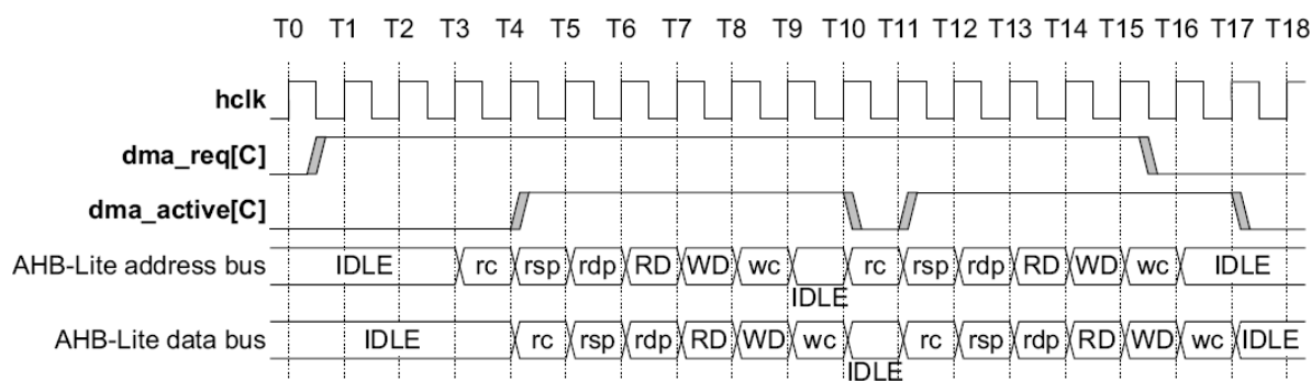
Рисунок 126 – Диаграмма работы при получении запроса на обработку по уровню
