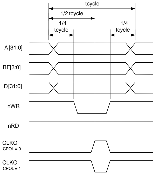
Рисунок 30 – Диаграмма записи
