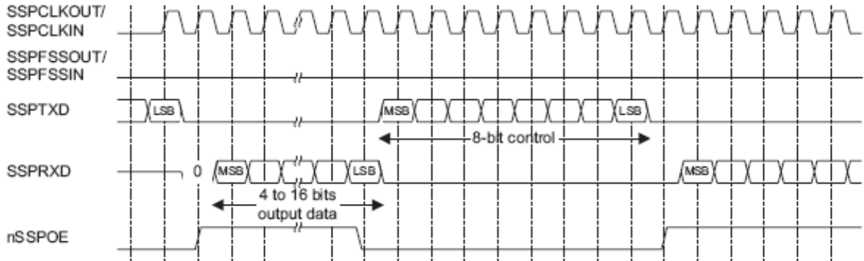
Рисунок 111 – Формат синхронного обмена протокола Microwire (непрерывный обмен)
