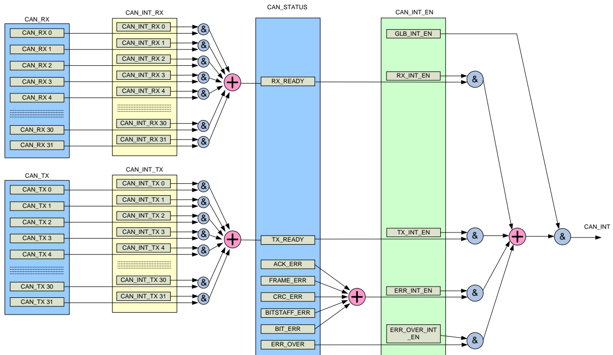
Рисунок 57 – Схема формирования прерывания блока CAN
