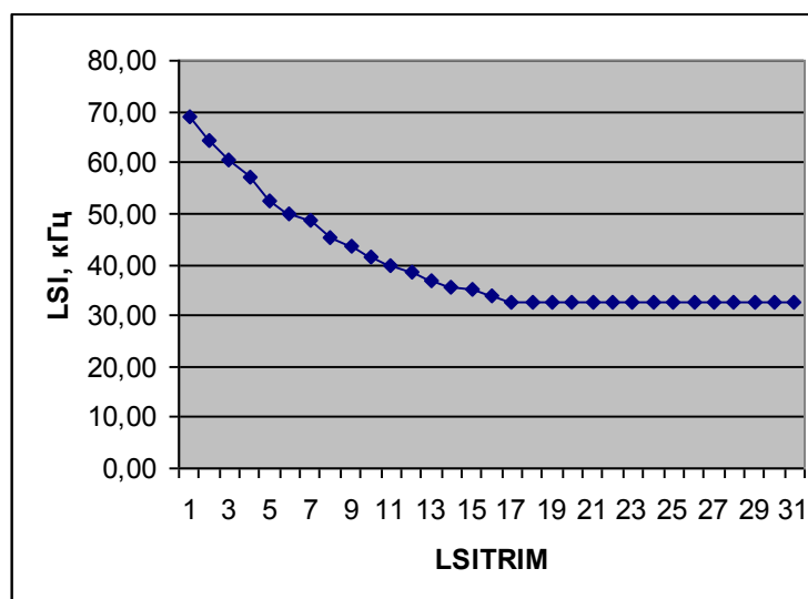
Рисунок 26 – Зависимость частоты LSI от значения LSITRIM
