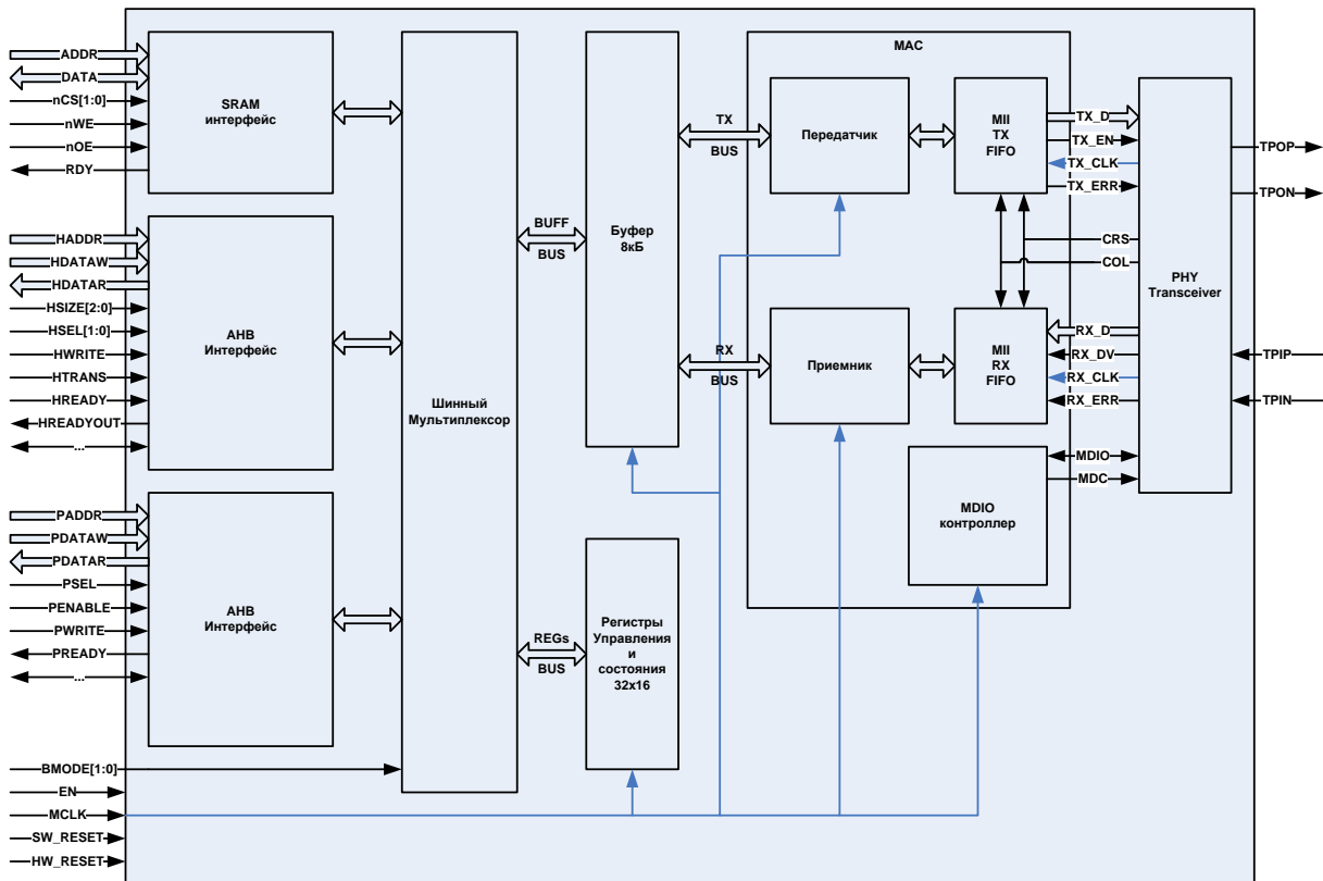
Рисунок 136 – Структурная схема контроллера интерфейса Ethernet
