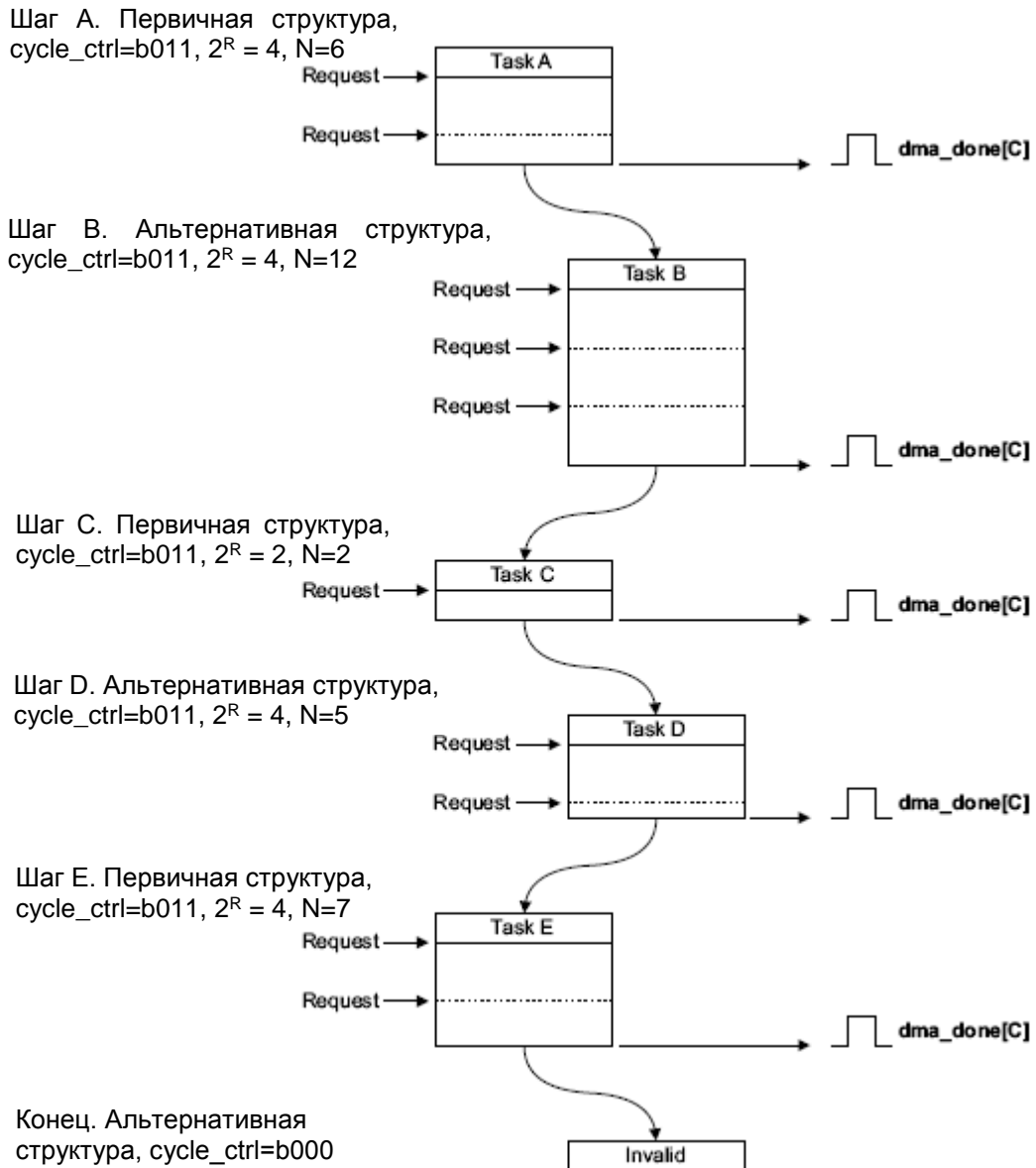
Рисунок 131 – Пример функционирования контроллера в режиме «пинг-понг»
