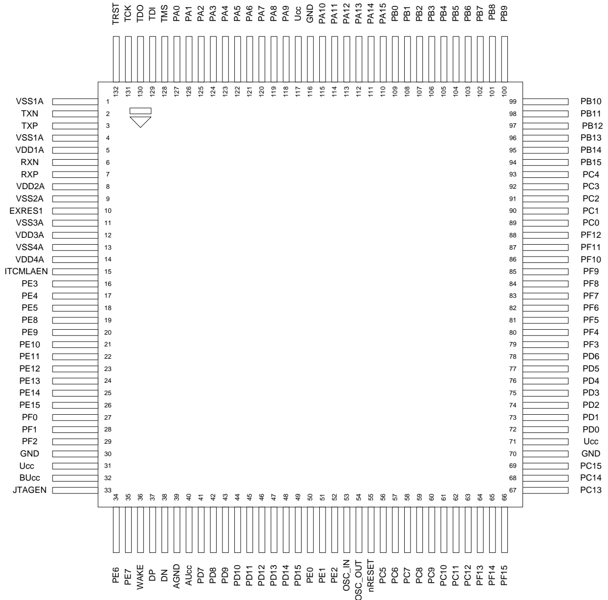
Рисунок 4 – 132-х выводной металлокерамический корпус 4229.132-3
