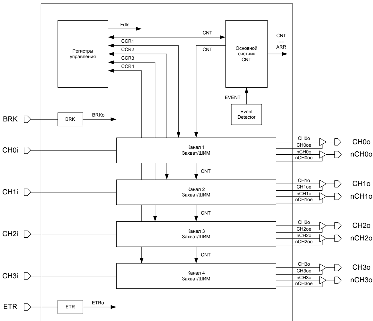
Рисунок 65 – Структурная схема таймера
