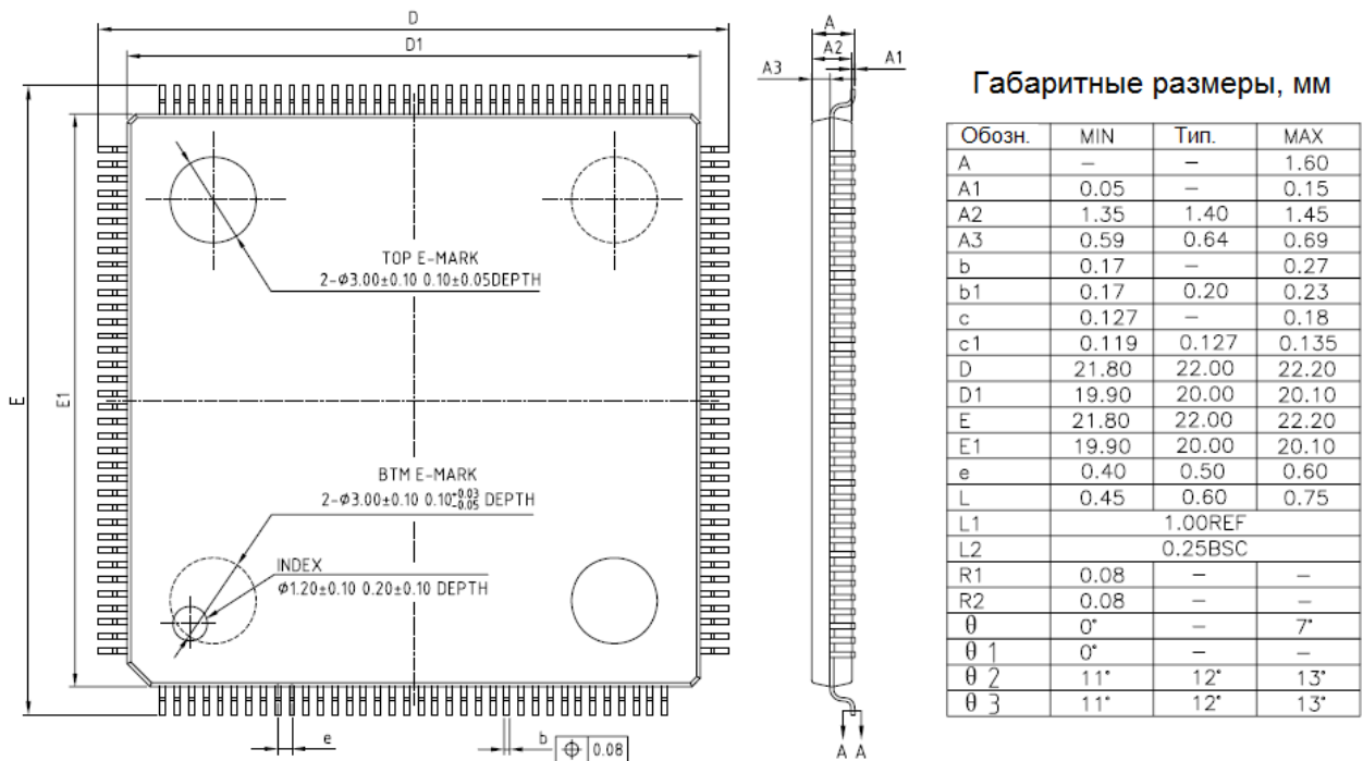
Рисунок 148 – Корпус LQFP144
