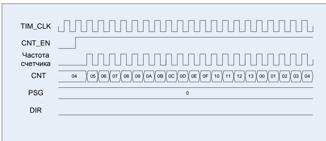
Рисунок 66 – Диаграммы работы таймера, счет вверх от 0 до 0x0013, стартовое значение 0x0004
