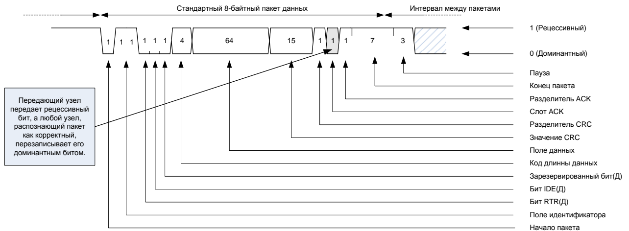
Рисунок 52 – Контроль подтверждения
