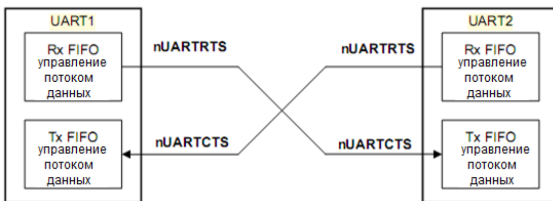
Рисунок 122 – Взаимодействие двух устройств последовательной связи с аппаратным управлением потоком данных
