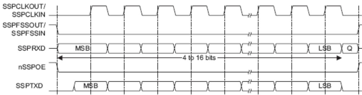
Рисунок 104 – Формат синхронного обмена протокола SPI, SPO=0, SPH=0 (одиночный обмен)
