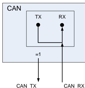
Рисунок 42 – Режим работы только на прием – Receive Only Mode
