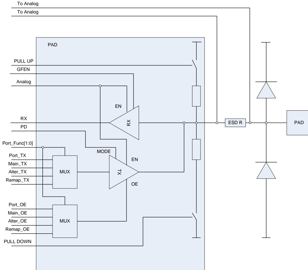
Рисунок 28 – Порты ввода/вывода
