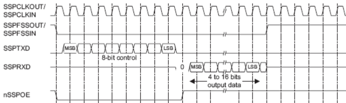
Рисунок 110 – Формат синхронного обмена протокола Microwire (одиночный обмен)
