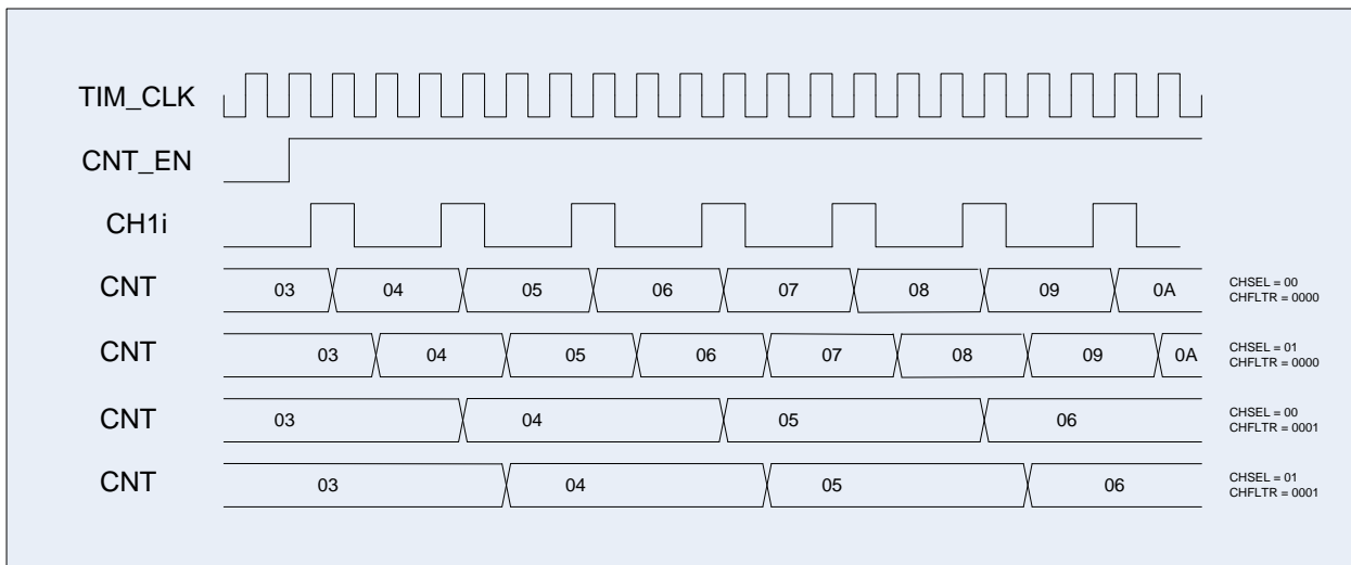
Рисунок 78 – Диаграмма внешнего тактирования с разными вариантами фильтра
