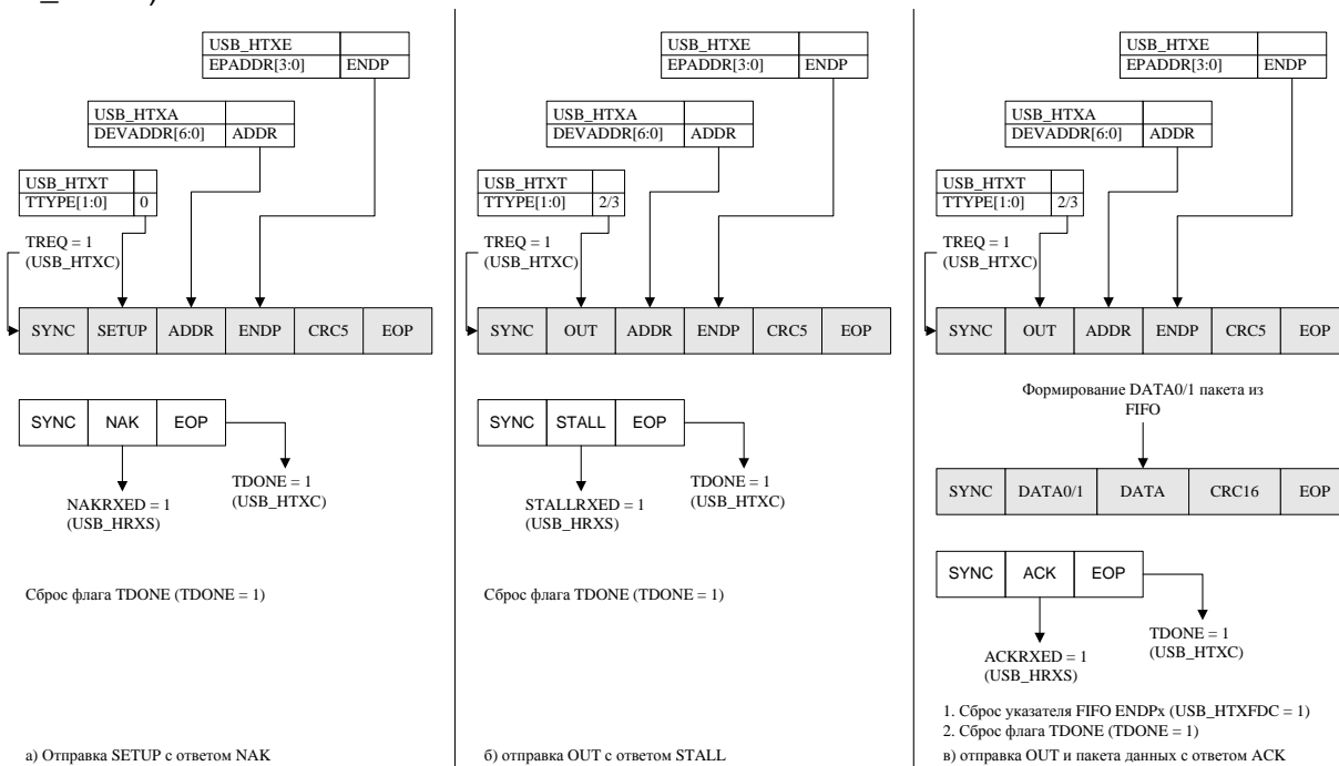
Рисунок 38 (а, б, в) – Транзакция SETUP/OUT (USB Host)
