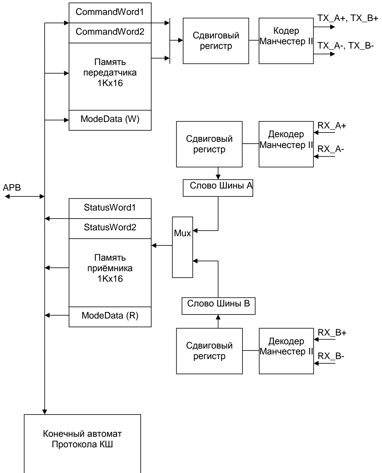
Рисунок 62 – Структурная схема работы в режиме КШ
