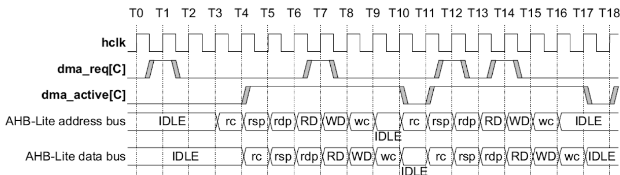
Рисунок 125 – Диаграмма работы при получении импульсного запроса от периферийного блока
