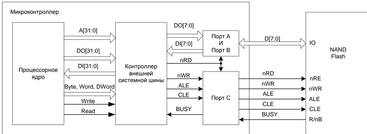
Рисунок 32 – Подключение внешней NAND Flash
