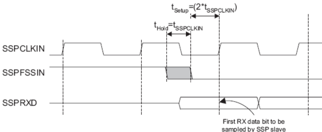
Рисунок 112 – Формат Microwire, требования к времени установки и удержания сигнала SSPFSSIN
