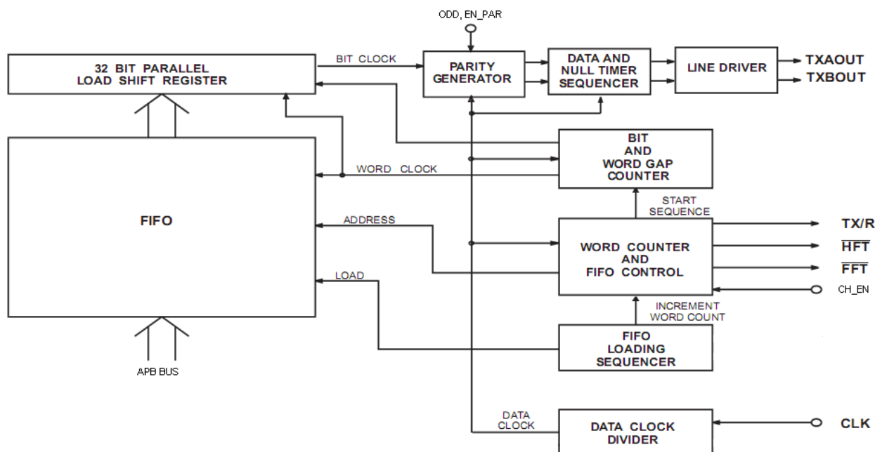
Рисунок 100 – Структурная схема канала передачи
