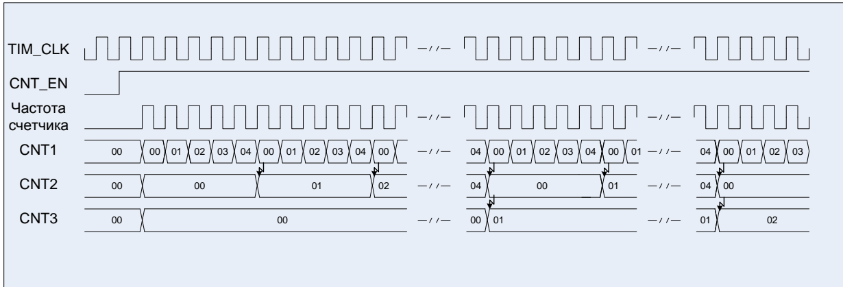
Рисунок 75 – Диаграммы работы трех таймеров в каскаде
