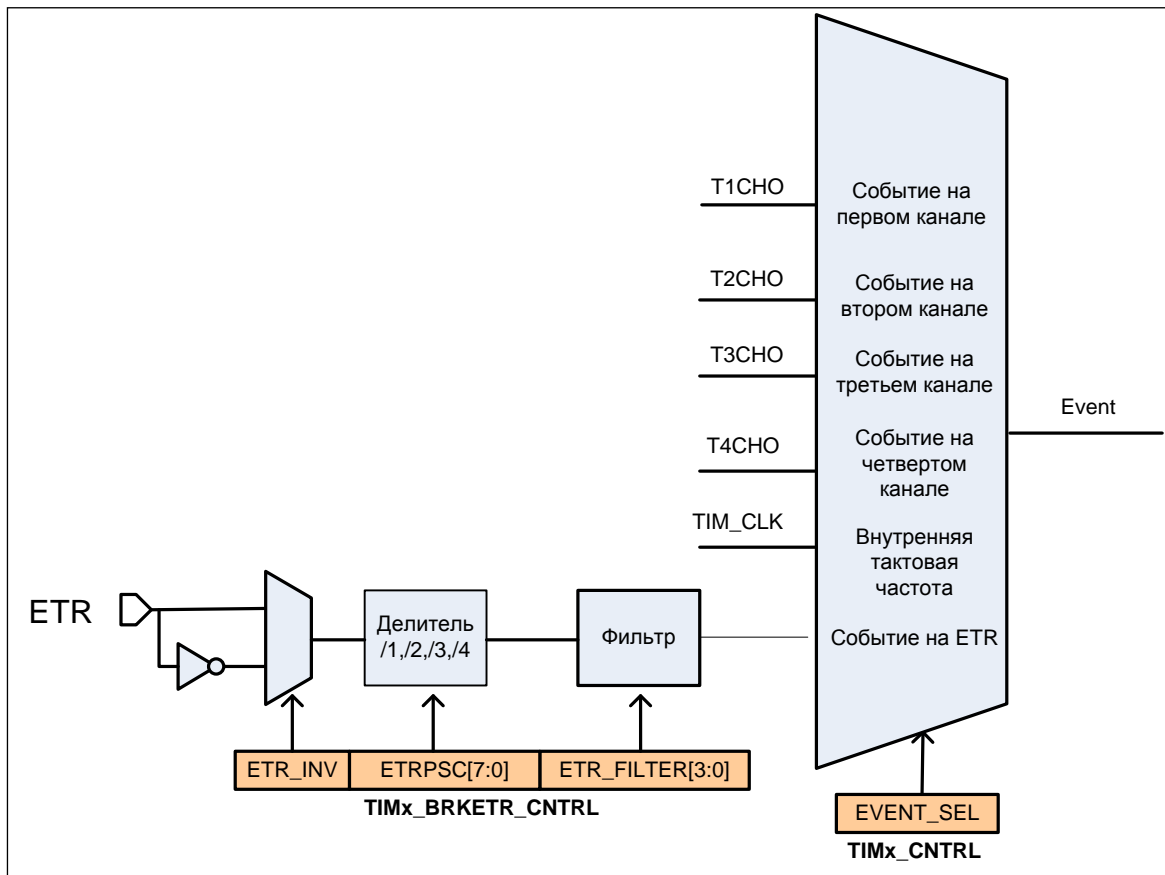
Рисунок 80 – Схема тактирования сигналом со входа ETR
