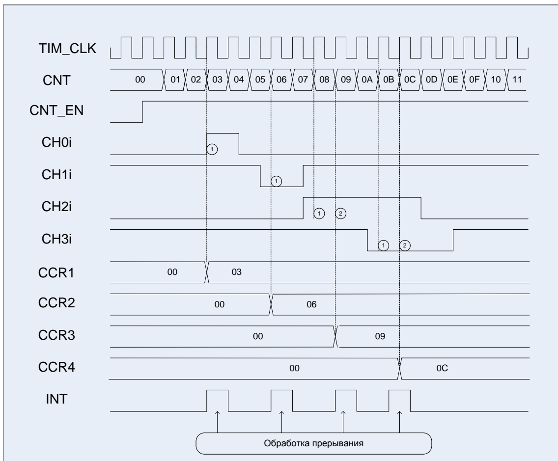
Рисунок 91 – Диаграммы примера работы в режиме захвата
