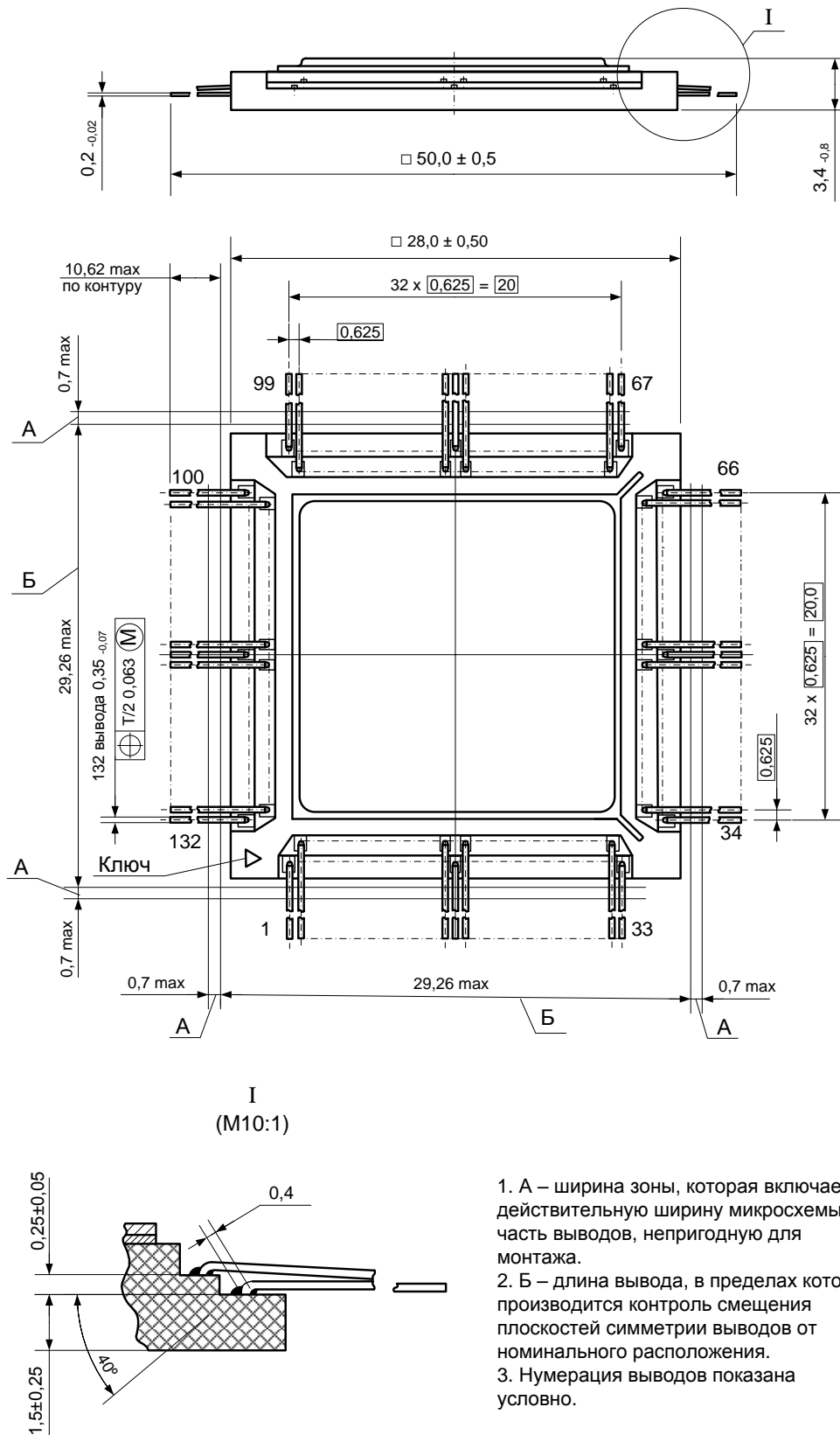
Рисунок 146 – Корпус 4229.132-3
