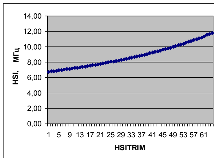
Рисунок 27 – Зависимость частоты HSI от значения HSITRIM
