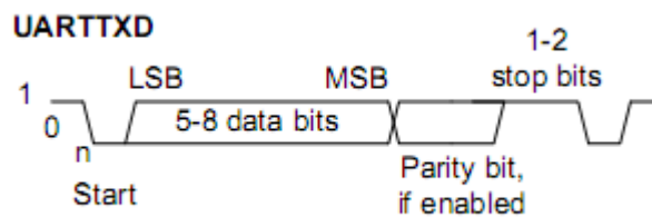
Рисунок 120 – Кадр передачи данных
