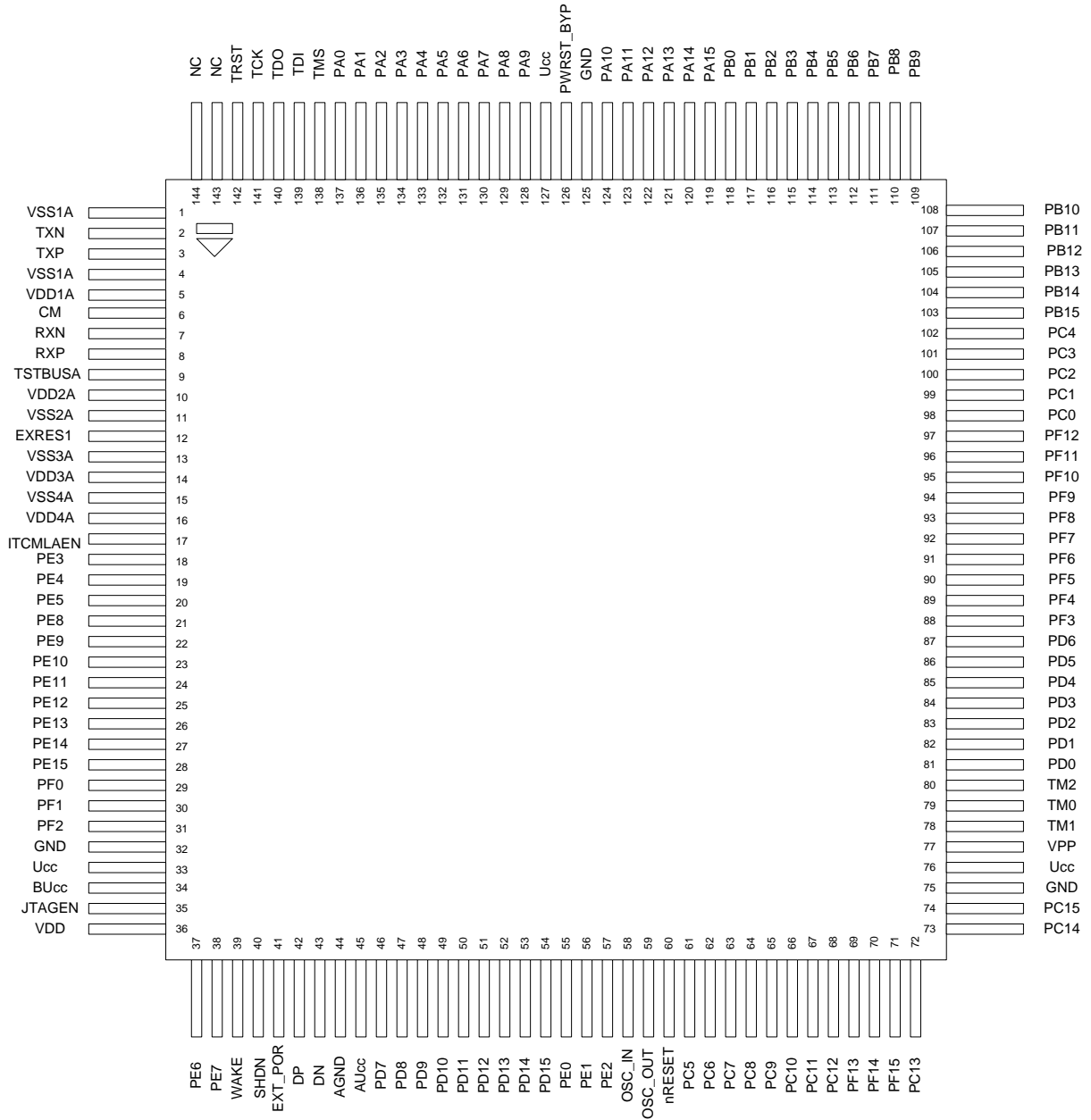
Рисунок 5 – 144-выводной пластиковый корпус LQFP144
