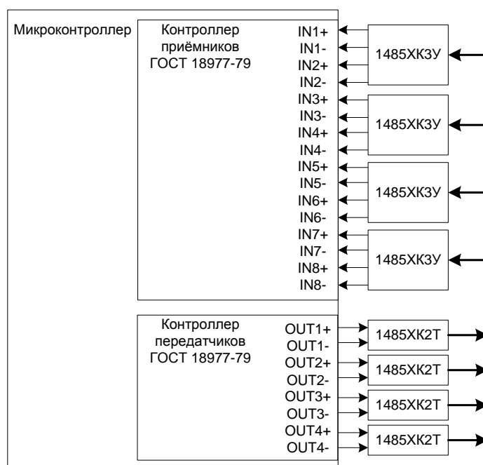
Рисунок 97 – Структура блока контроллера интерфейса по ГОСТ 18977-79
