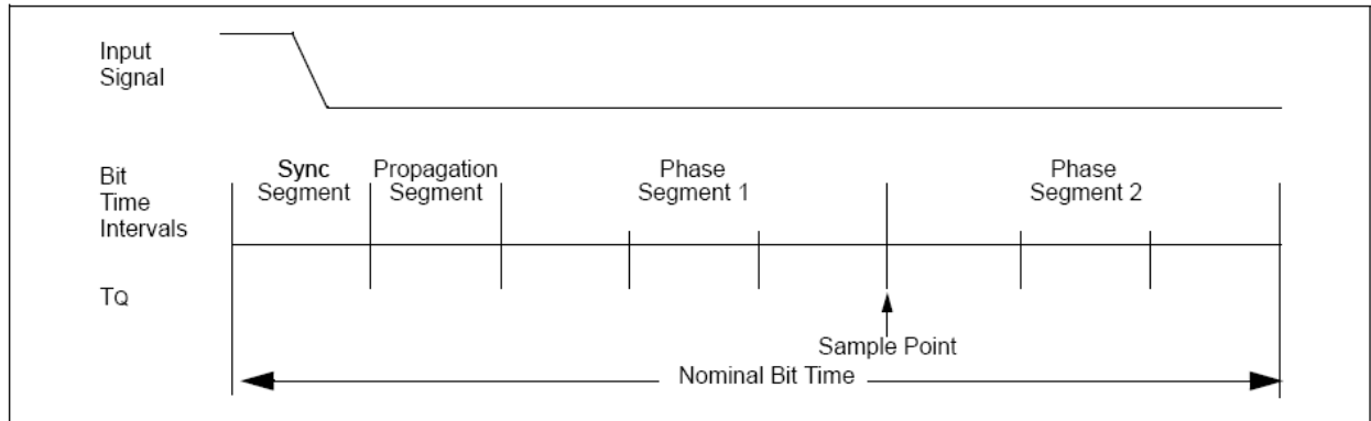
Рисунок 50 – Структура битового интервала
