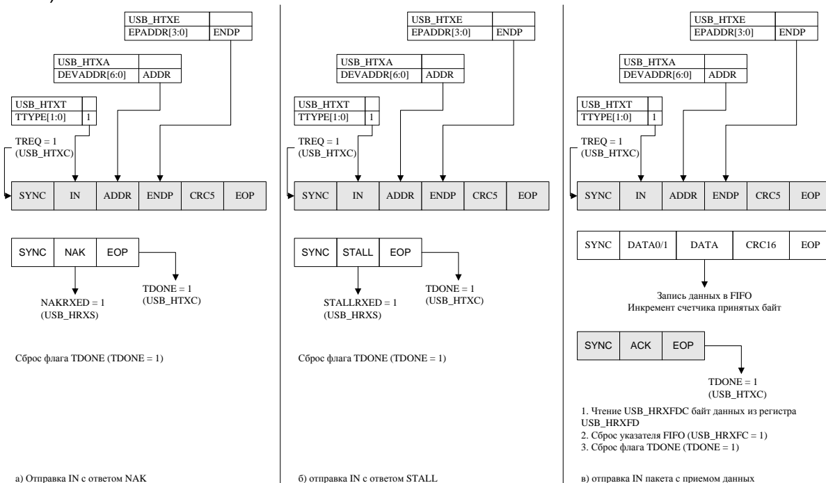
Рисунок 39 (а, б, в) – Транзакция IN (USB Host)
