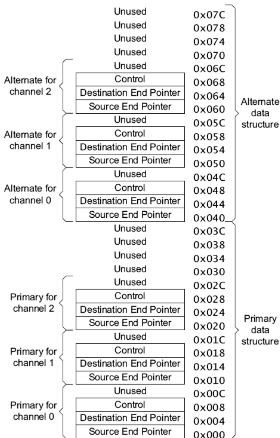
Рисунок 135 – Карта памяти для трех каналов DMA, включая альтернативную структуру управляющих данных (где Destination end pointer – указатель конца данных приемника; Source end pointer – указатель конца данных источника; Control – управление)
