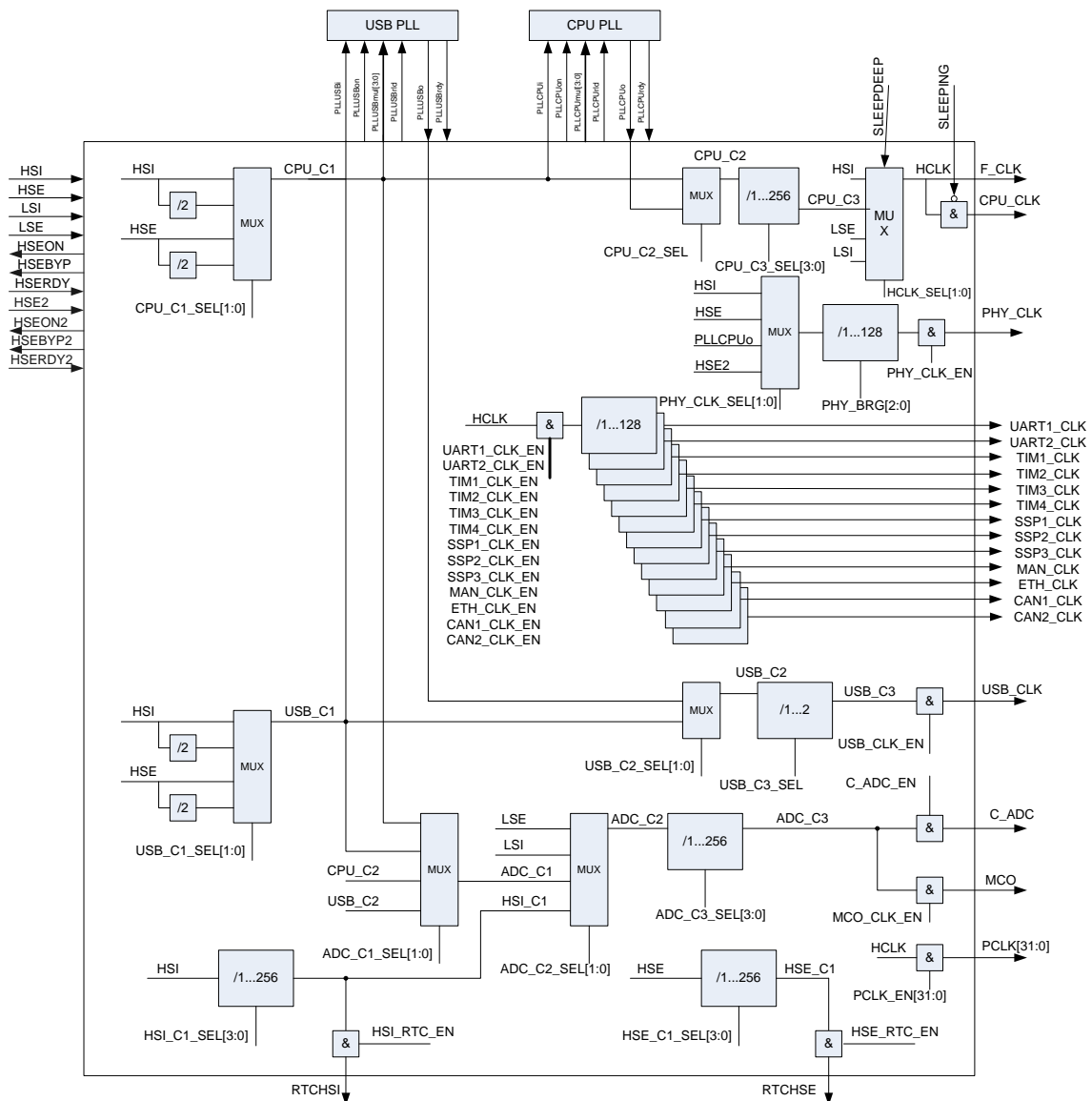
Рисунок 24 – Структурная блок-схема формирования тактовой частоты
