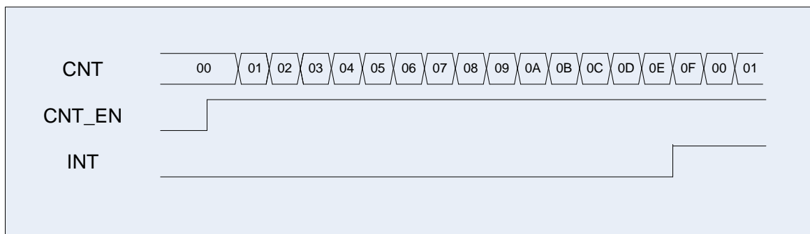
Рисунок 90 – Режим обычного счетчика
