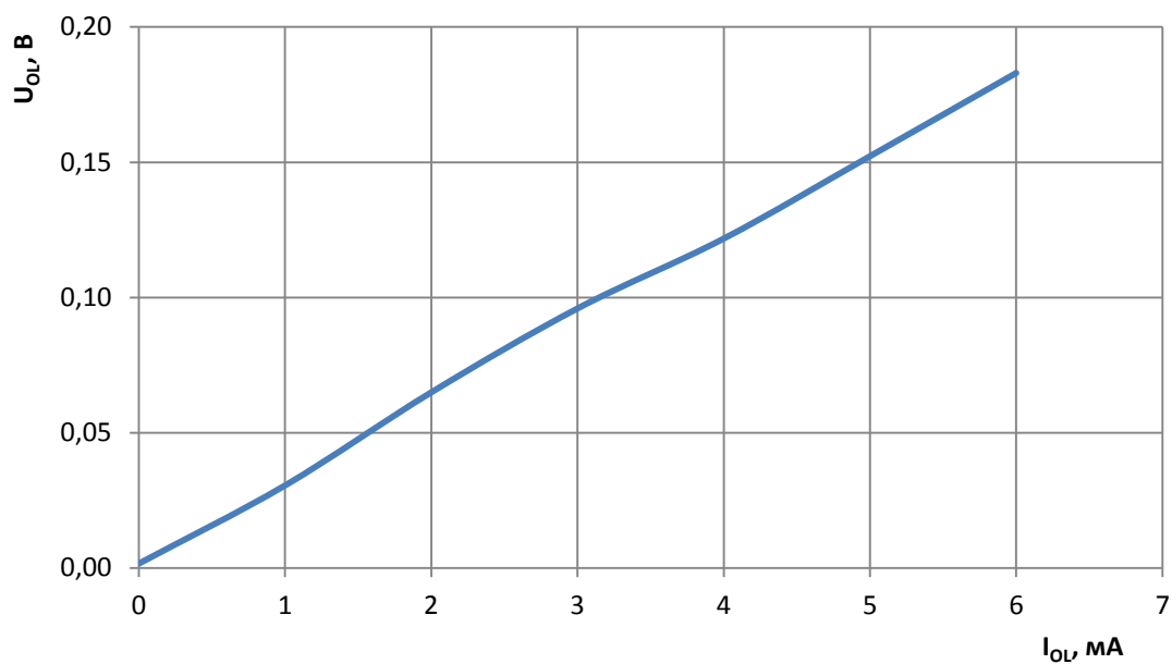
Рисунок 145 – Зависимость выходного напряжения низкого уровня от выходного тока низкого уровня при напряжении питания 3,0 В
