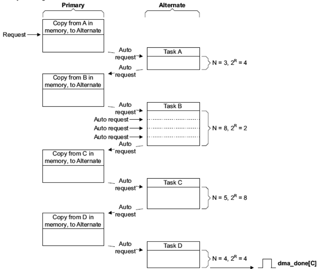
Рисунок 132 – Пример работы DMA в режиме с «Исполнением с изменением конфигурации»
