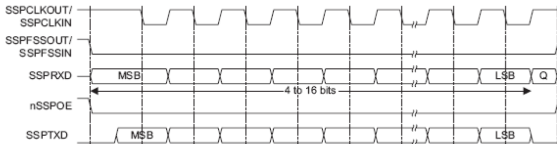
Рисунок 107 – Формат синхронного обмена протокола SPI, SPO=1, SPH=0 (одиночный обмен)
