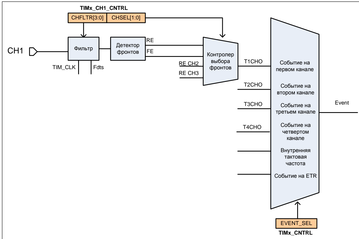
Рисунок 77 – Тактирование с входа первого канала
