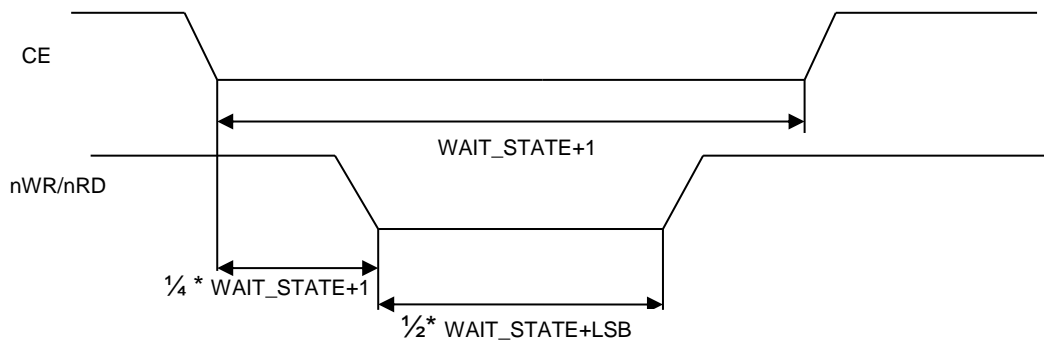
Рисунок 33 – Длительность фаз обращения в тактах процессора
