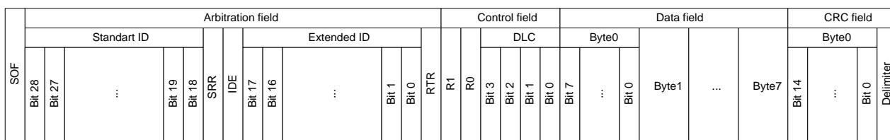
Рисунок 47 – Структура расширенного пакета данных
