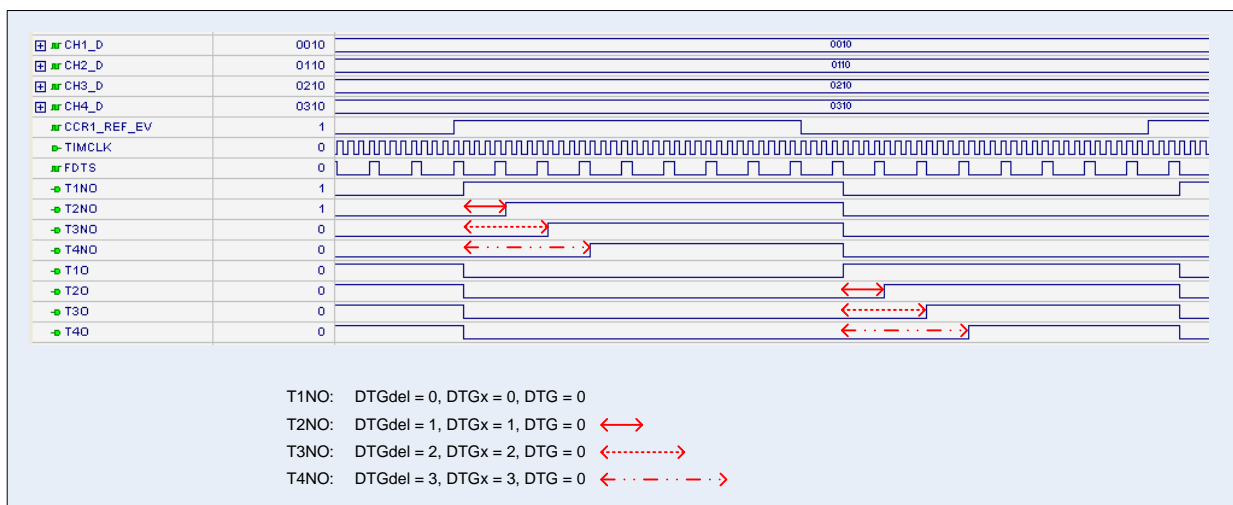
Рисунок 88 – Диаграмма работы схемы DTG
