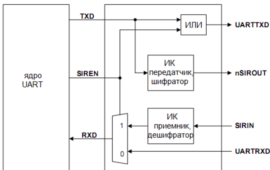
Рисунок 118 – Структурная схема кодека IrDA
