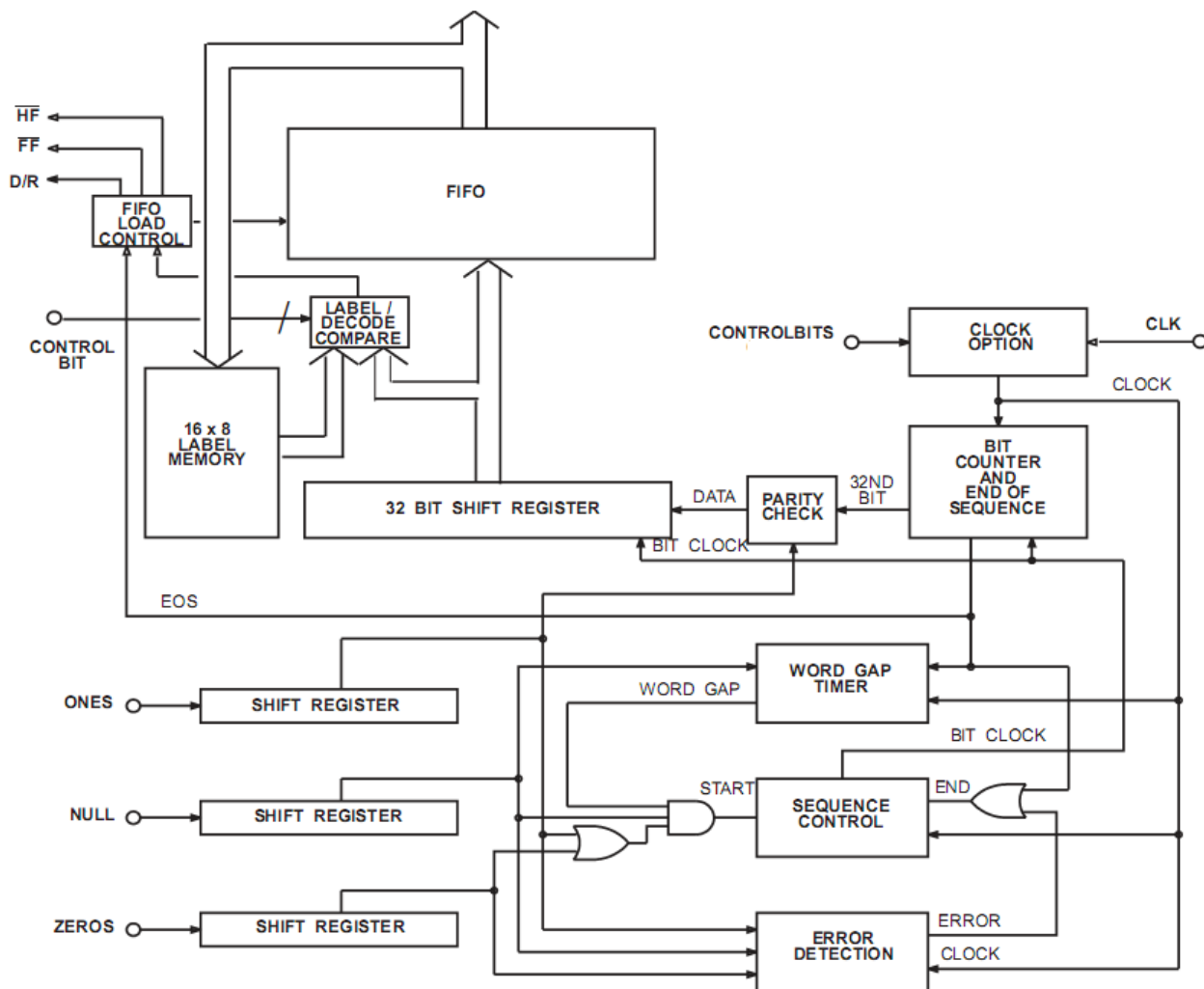
Рисунок 99 – Структурная схема канала приёма
