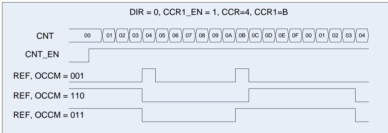
Рисунок 89 – Диаграмма работы схемы в режиме ШИМ, CCR1_EN = 1
