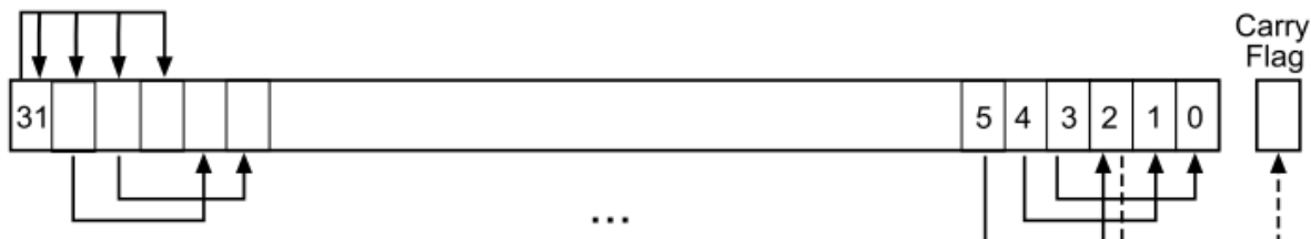
Рисунок 20 – Инструкция ASR # 3
