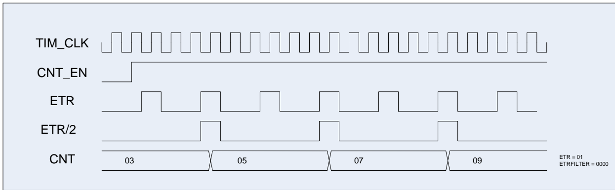
Рисунок 81 – Диаграмма тактирования сигналом со входа ETR
