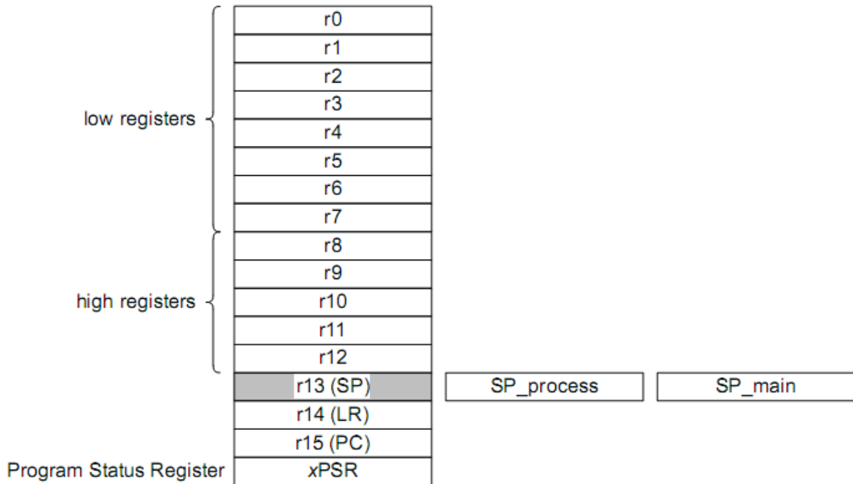
Рисунок 19 – Регистры ядра
