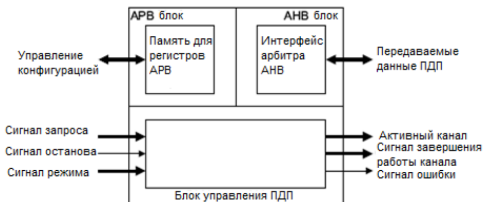
Рисунок 124 – Структурная схема контроллера
