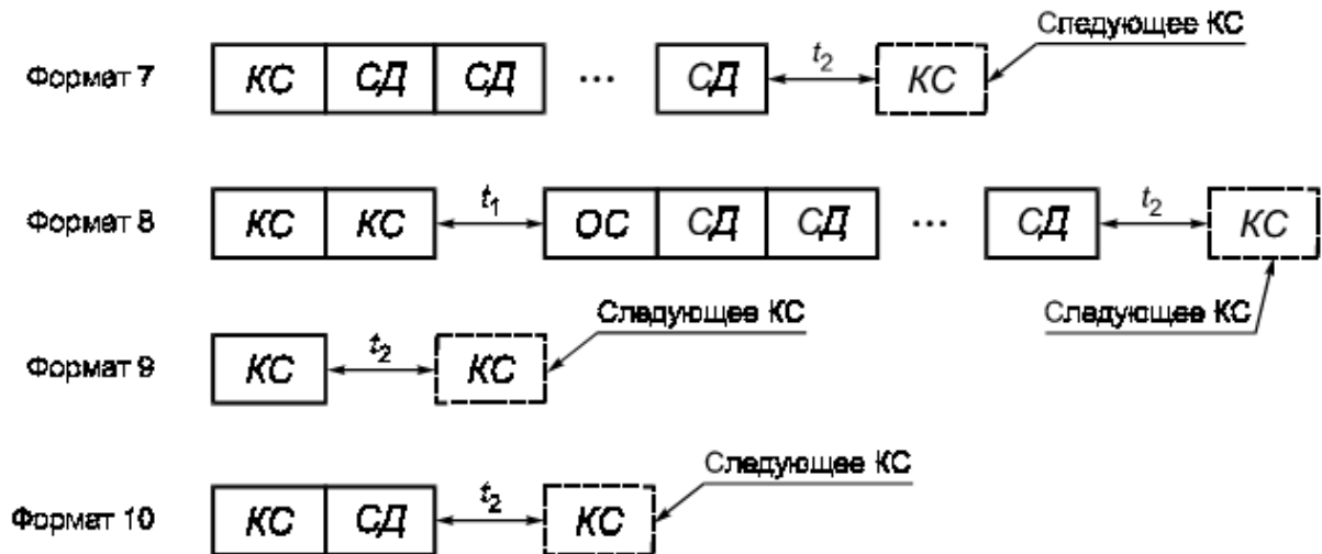
Рисунок 60 – Форматы групповых сообщений
