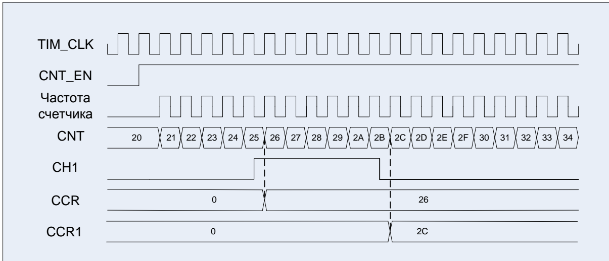
Рисунок 83 – Диаграмма захвата события со входа первого канала
