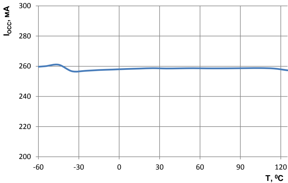
Рисунок 141 – Зависимость динамического тока потребления от температуры при: f_C = 144 МГц
