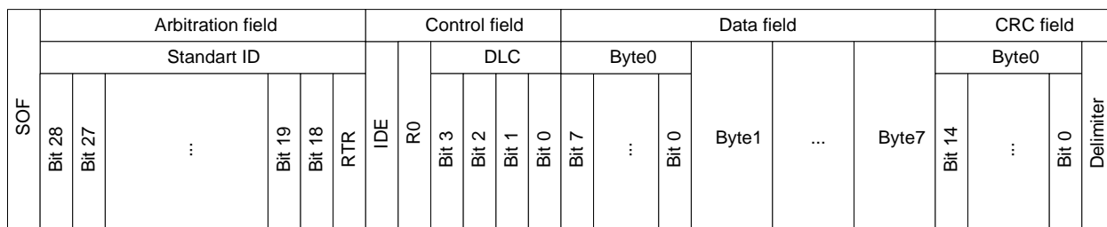
Рисунок 46 – Структура стандартного пакета данных
