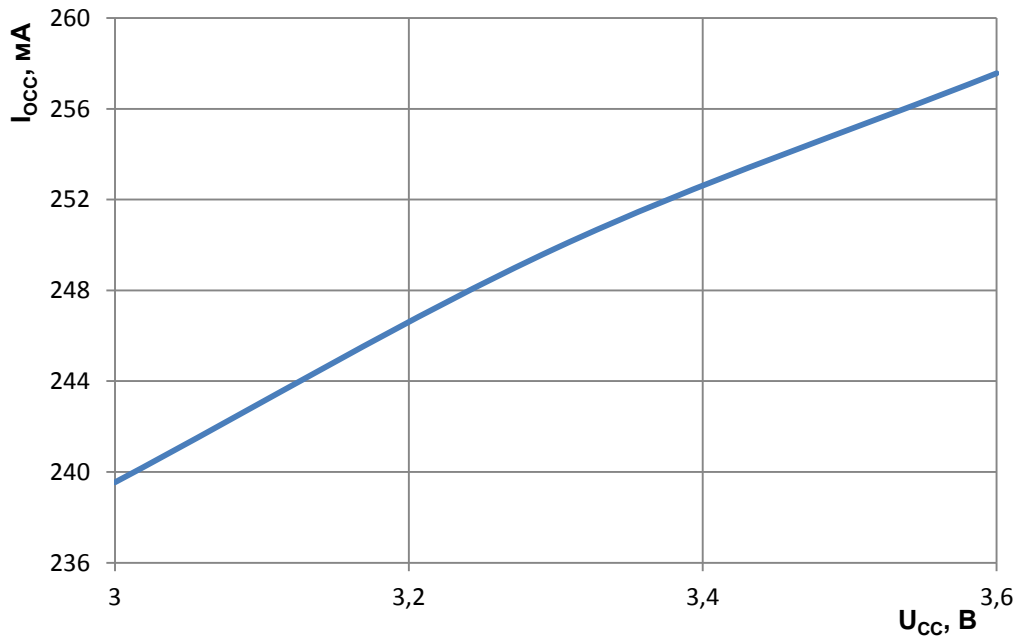
Рисунок 142 – Зависимость динамического тока потребления от напряжения питания
