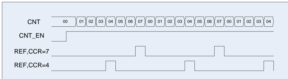
Рисунок 85 – Диаграмма работы схемы в режиме ШИМ, CCR1_EN=0
