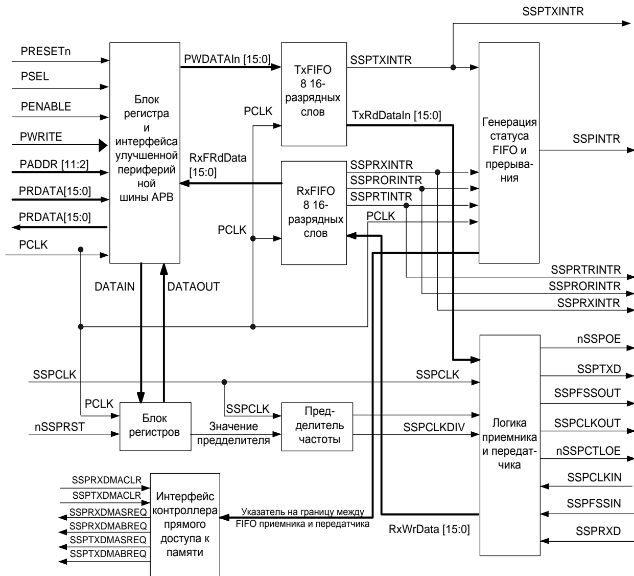
Рисунок 101 – Структурная схема модуля SSP
