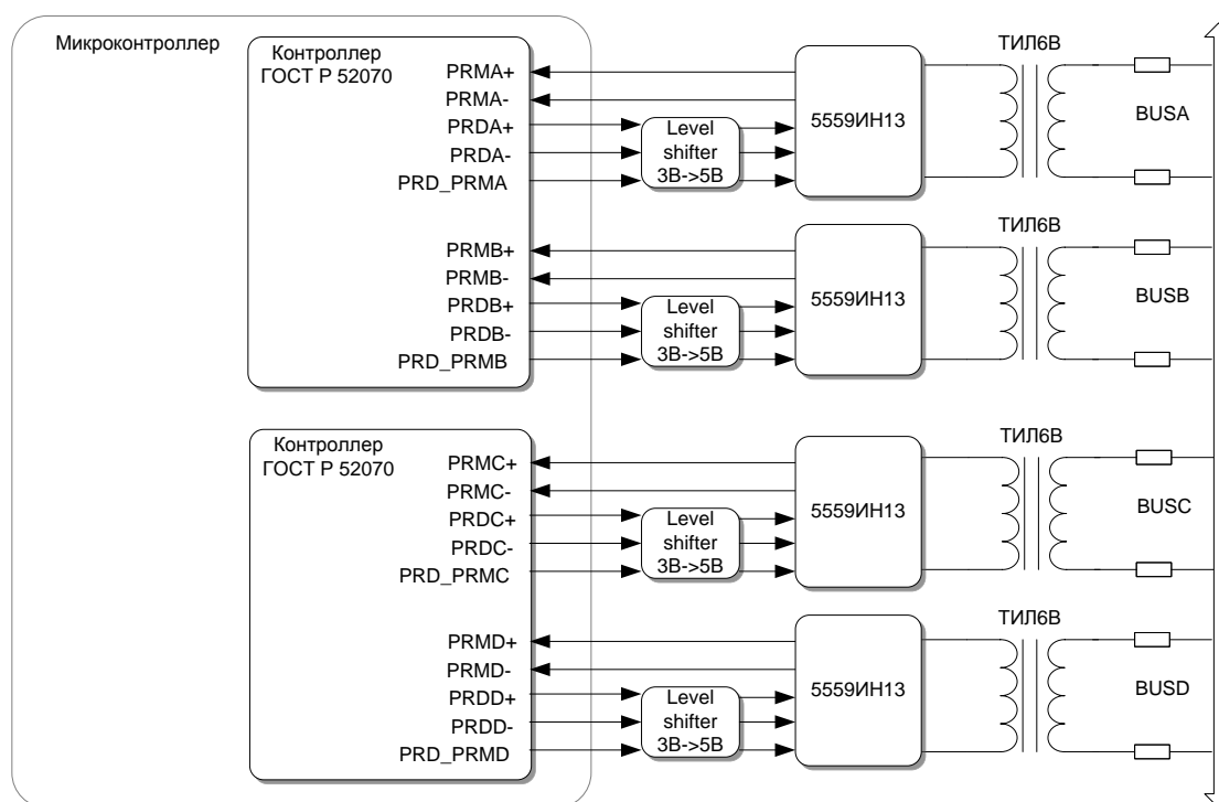
Рисунок 58 – Структурная схема контроллера интерфейса по ГОСТ Р 52070-2003
