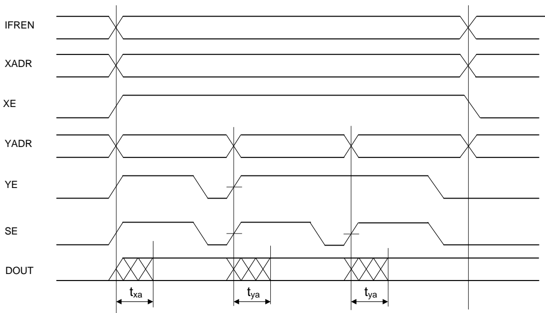
Рисунок 17 – Временная диаграмма чтения памяти
