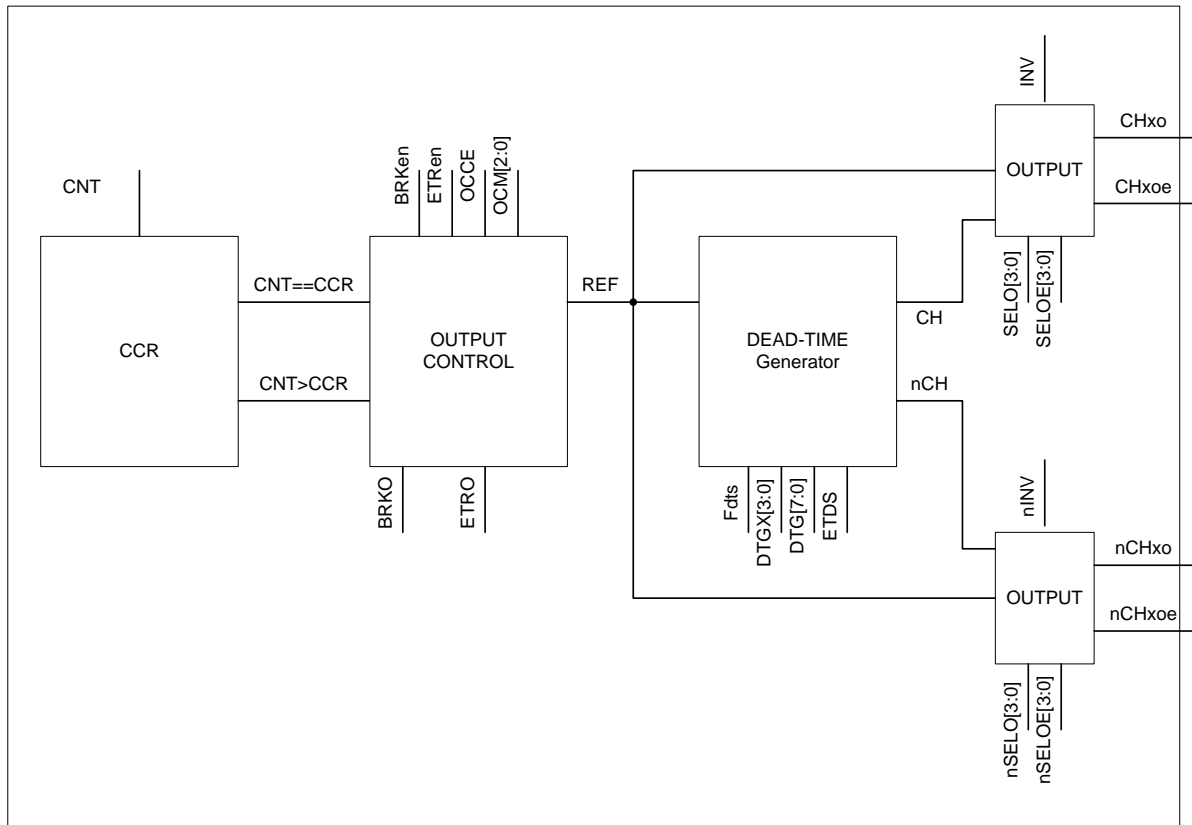
Рисунок 84 – Структурная схема блока сравнения
