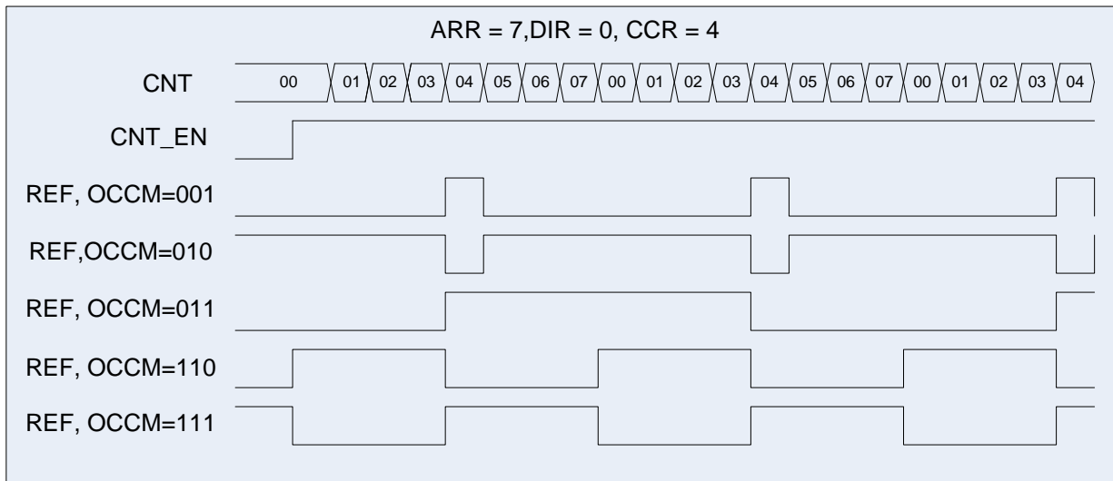
Рисунок 86 – Диаграмма работы схемы в режиме ШИМ, CCR1_EN=0
