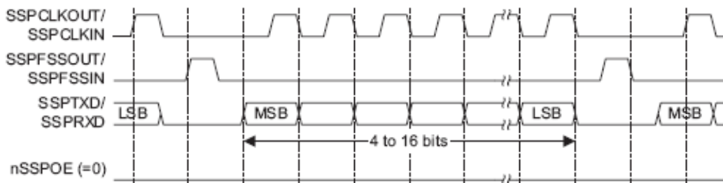
Рисунок 105 – Формат синхронного обмена протокола SPI, SPO=0, SPH=0 (непрерывный обмен)
