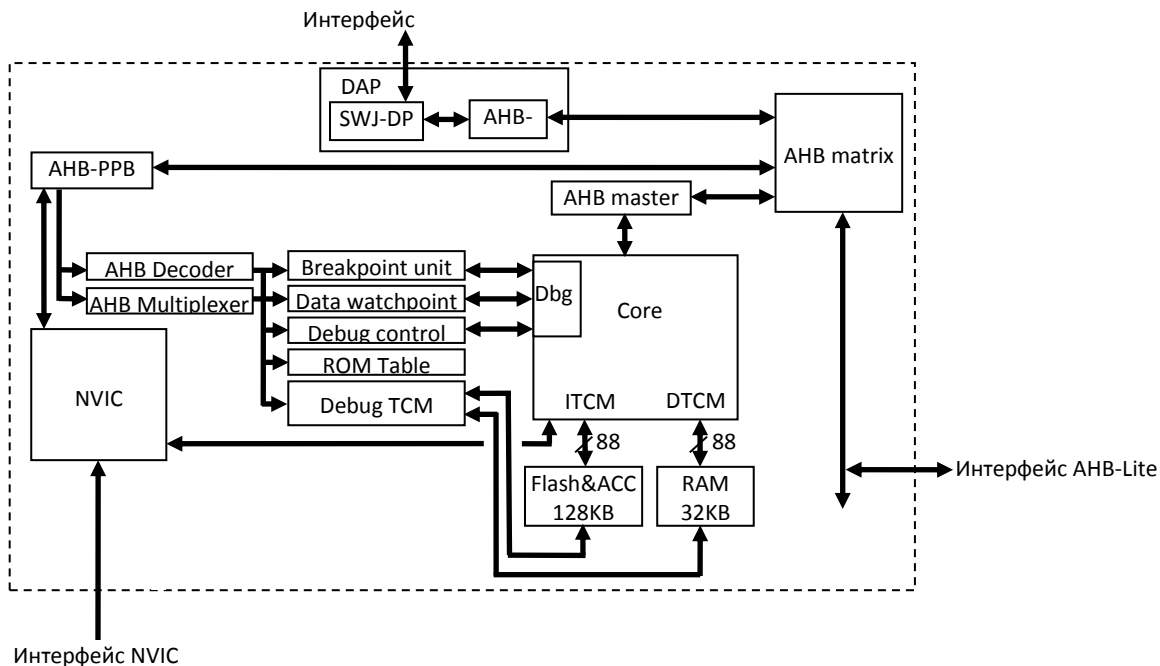
Рисунок 18 – Структурная блок-схема процессорного ядра
