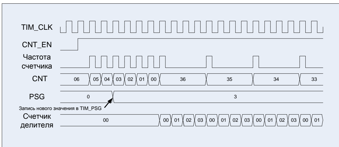
Рисунок 72 – Диаграммы работы счетчика: счет вниз (CNT_MODE = 00, EVENT_SEL = 0000, DIR = 1)
