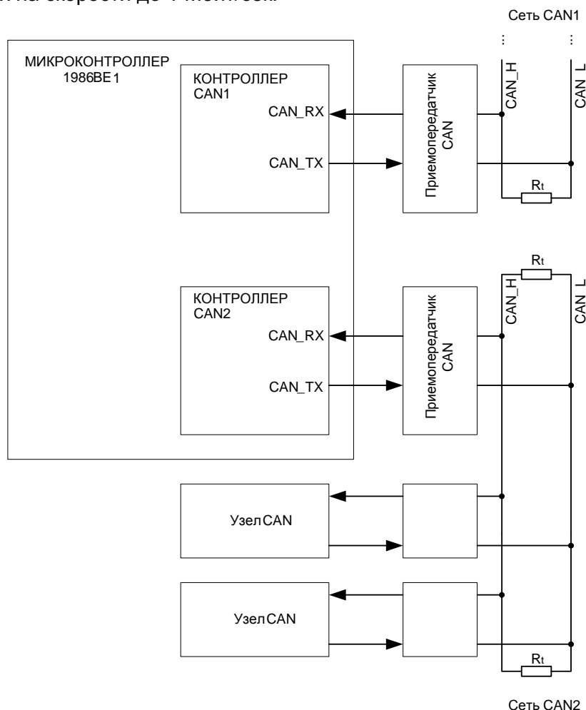
Рисунок 40 – Структурная блок – схема организации сети CAN
