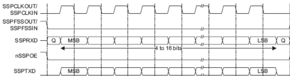
Рисунок 106 – Формат синхронного обмена протокола SPI, SPO=0, SPH=1
