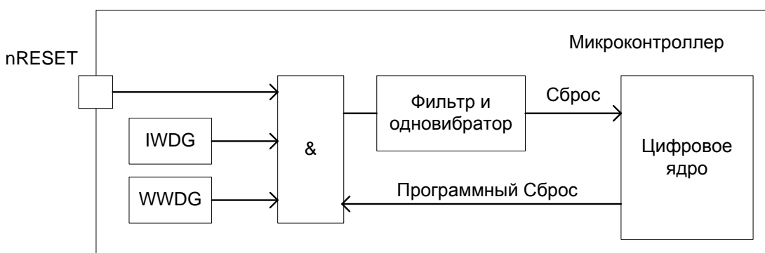
Рисунок 8 – Структурная блок-схема сброса
