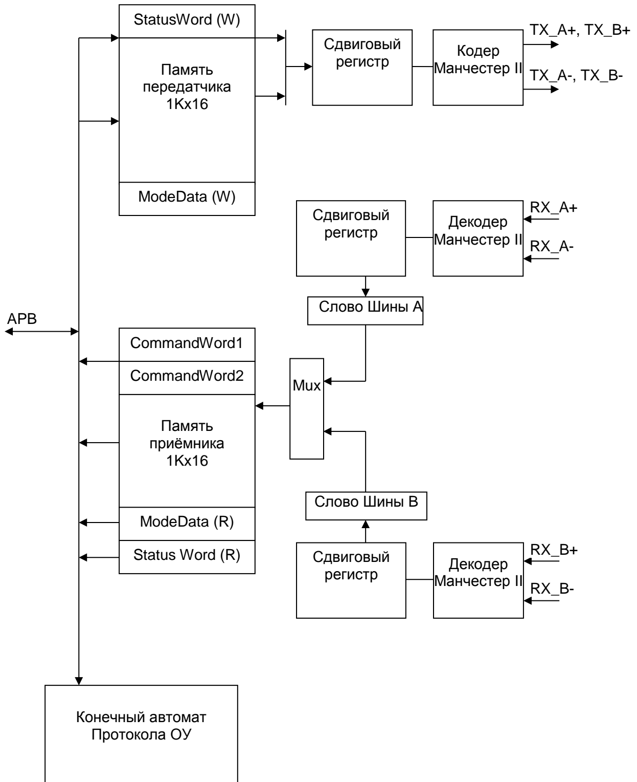
Рисунок 63 – Структурная схема работы в режиме ОУ
