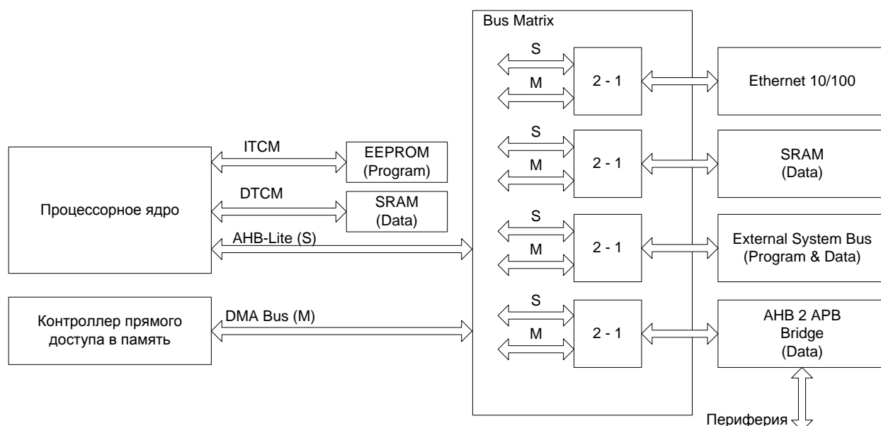
Рисунок 10 – Структурная схема организации памяти
