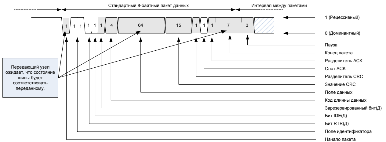
Рисунок 54 – Контроль передаваемых бит
