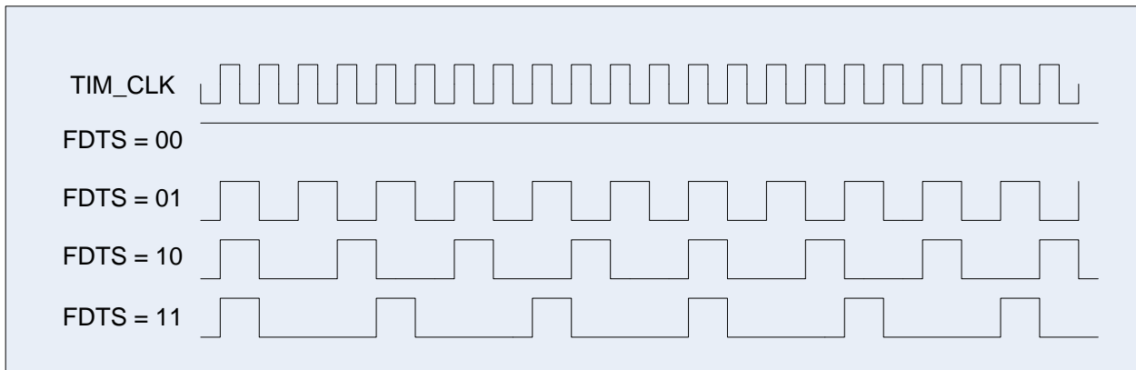
Рисунок 76 – Диаграммы возможных частот семплирования данных (FDTs)
