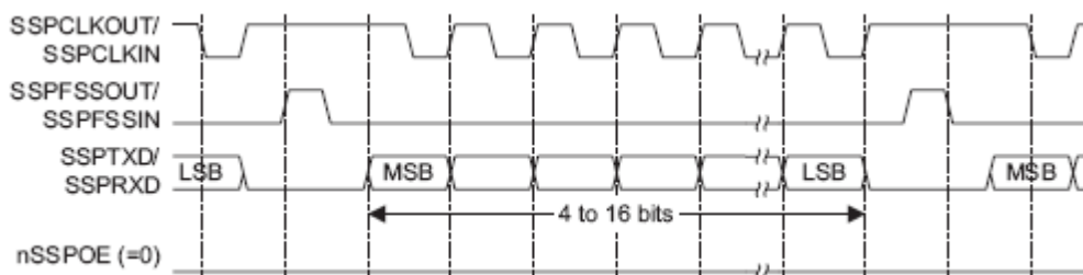
Рисунок 108 – Формат синхронного обмена протокола SPI, SPO=1, SPH=0 (непрерывный обмен)
