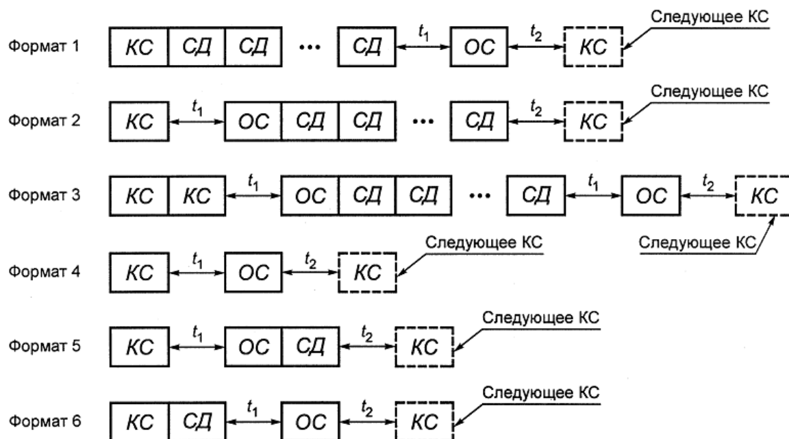
Рисунок 59 – Форматы сообщений
