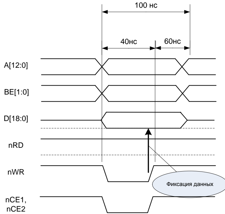
Рисунок 34 – Временная диаграмма цикла записи
