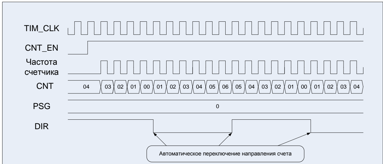
Рисунок 73 – Диаграммы работы счетчика: счет вниз/вверх (CNT_MODE = 01, EVENT_SEL = 0000, DIR = 1)
