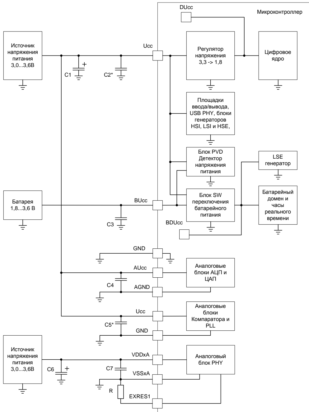
Рисунок 6 – Структурная блок-схема подачи питания
