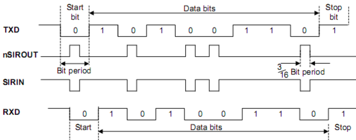
Рисунок 121 – Модуляция данных IrDA
