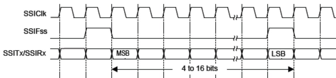
Рисунок 103 – Формат синхронного обмена протокола SSI (непрерывный обмен)
