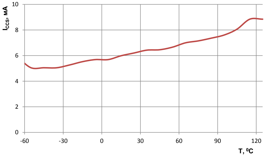
Рисунок 143 – Зависимость статического тока потребления в режиме покоя (регулятор напряжения выключен) от температуры при разном напряжении
