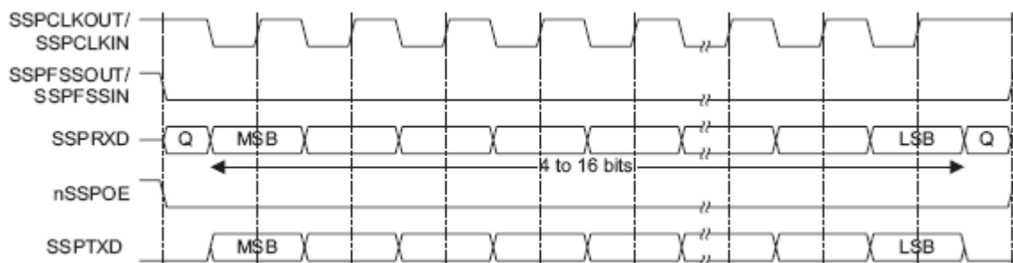
Рисунок 109 – Формат синхронного обмена протокола SPI, SPO=1, SPH=1
