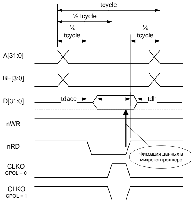
Рисунок 31 – Диаграмма чтения
