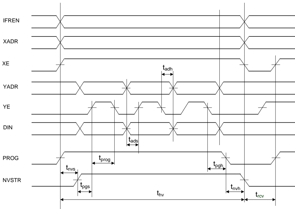
Рисунок 16 – Временная диаграмма записи памяти
