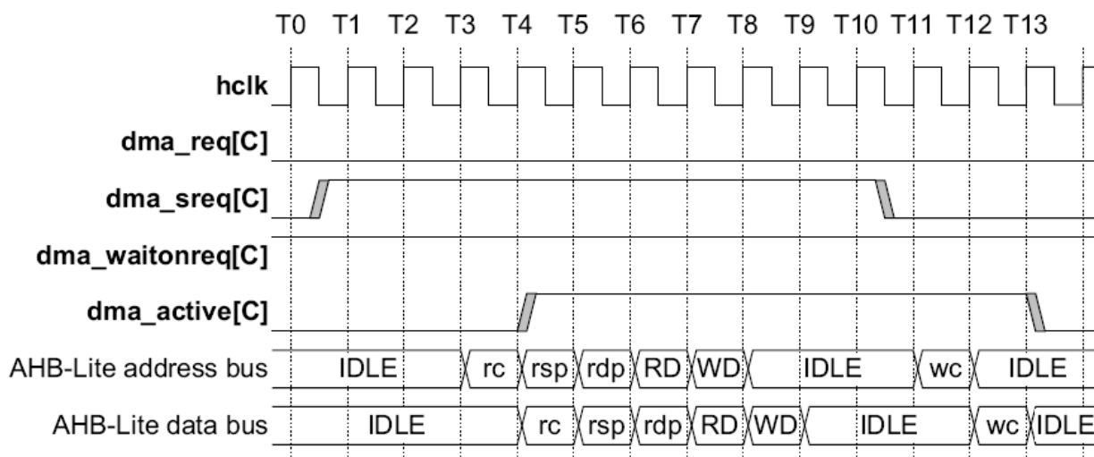
Рисунок 129 – Работа DMA при использовании dma_waitonreq совместно с dma_sreq
