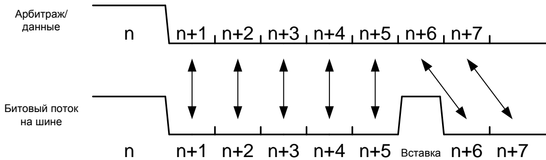
Рисунок 55 – Битстаффинг
