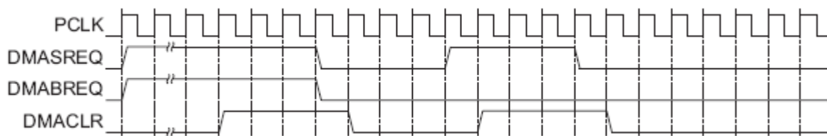
Рисунок 116 – Временные диаграммы обмена в режиме DMA
