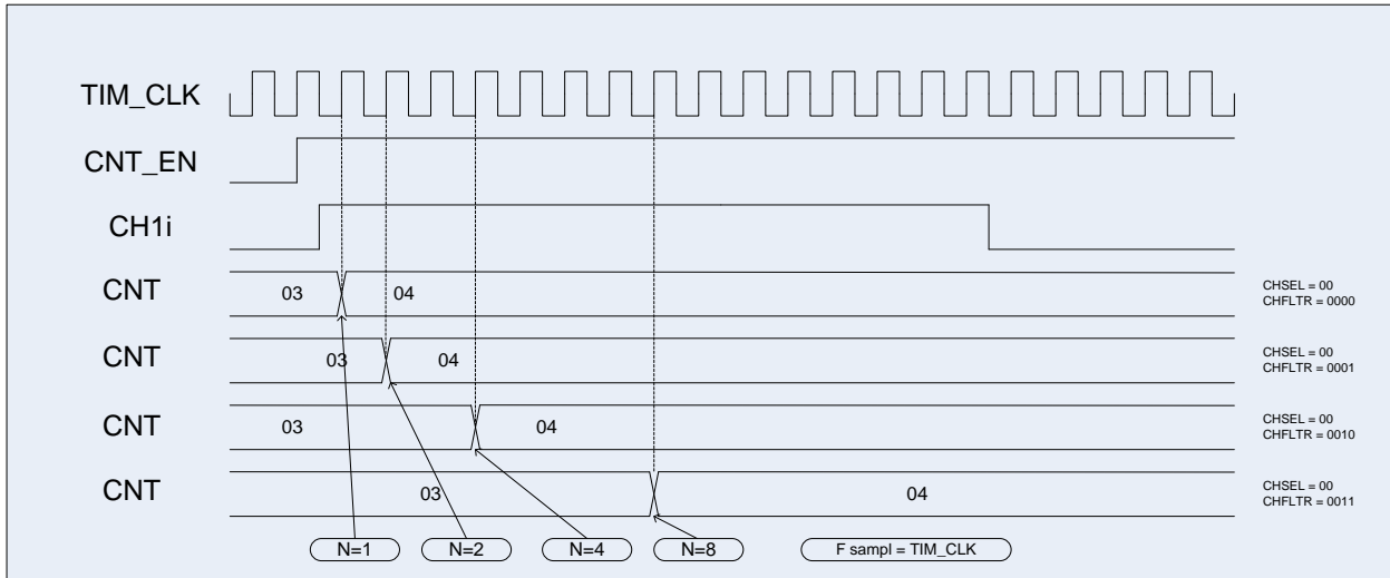
Рисунок 79 – Диаграмма внешнего тактирования с разными вариантами фильтра
