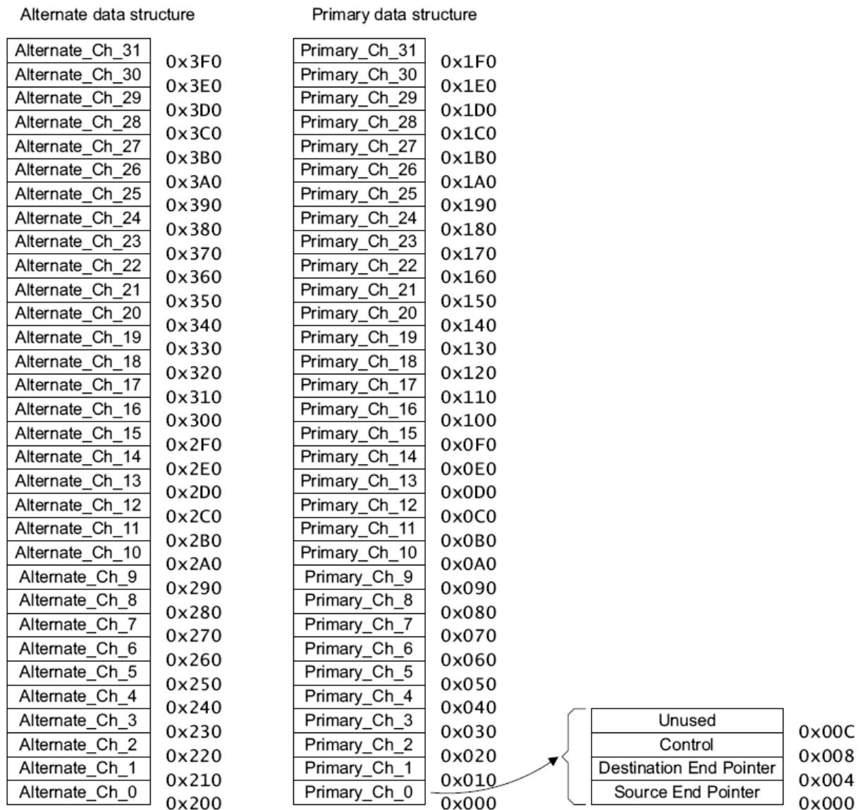
Рисунок 134 – Карта памяти для 32-х каналов, включая альтернативную структуру управляющих данных
