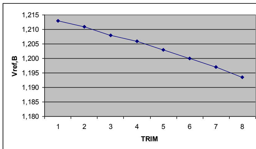
Рисунок 94 – Зависимость источника опорного напряжения от подстройки
