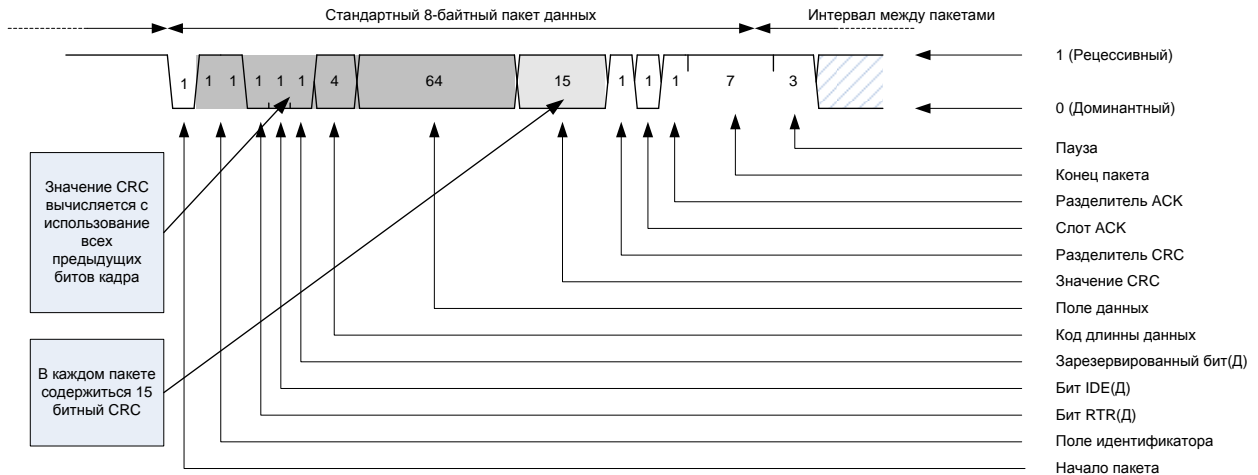
Рисунок 53 – Контроль CRC
