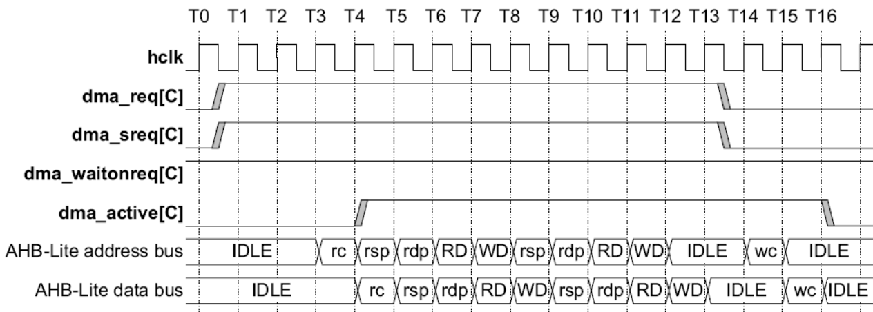
Рисунок 128 – Диаграмма работы контроллера DMA при использовании dma_waitonreq
