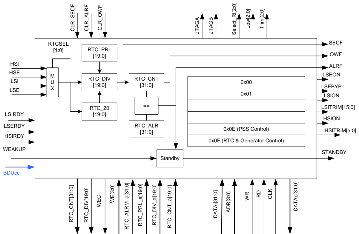
Рисунок 25 – Структурная блок-схема батарейного домена и часов реального времени
