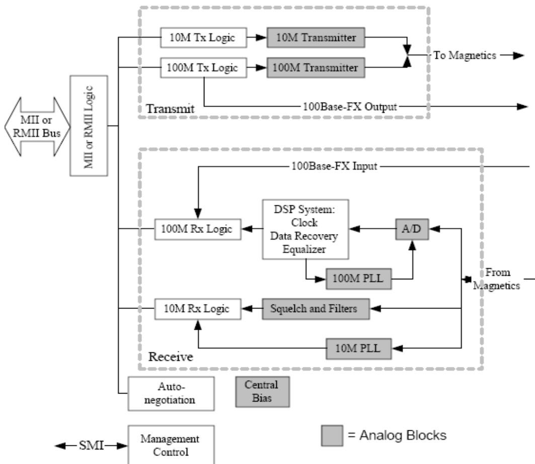
Рисунок 137 – Структурная схема модуля PHY
