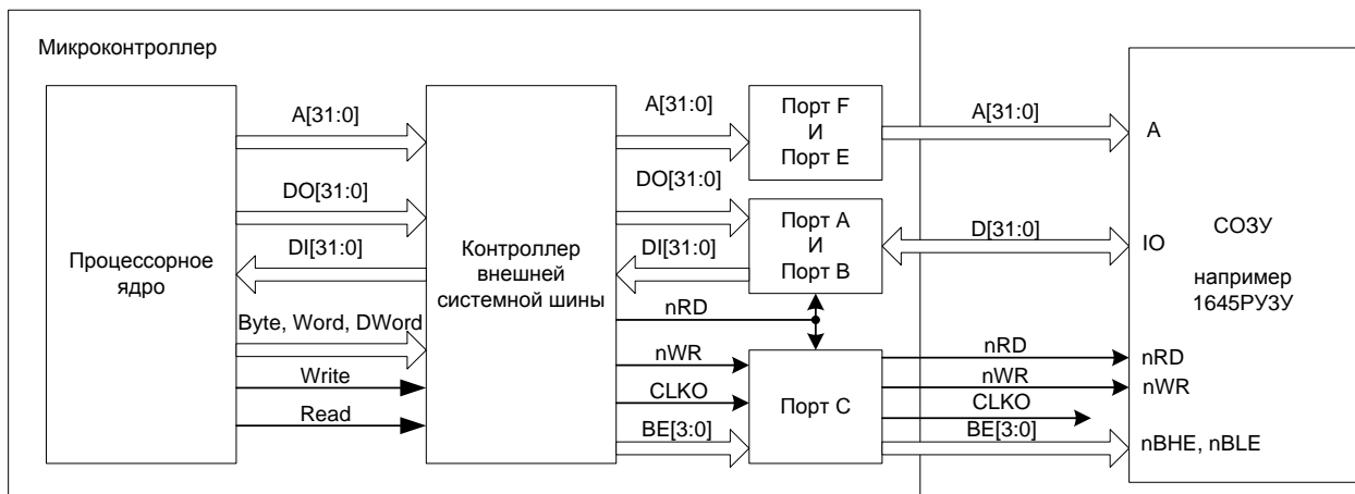
Рисунок 29 – Обмен по внешней системной шине
