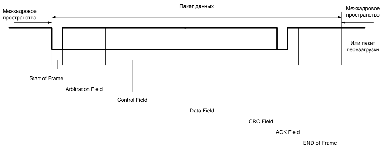
Рисунок 45 – Пакет сообщения CAN
