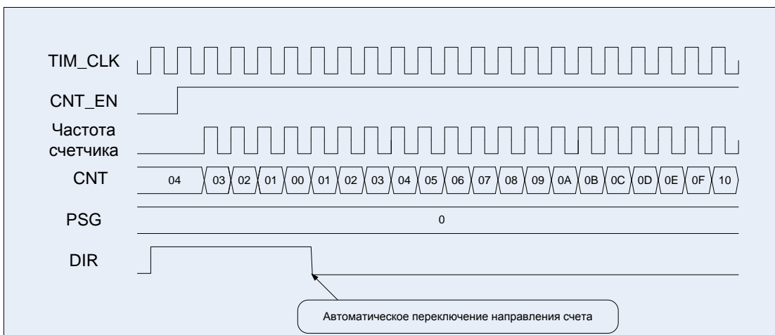
Рисунок 69 – Диаграммы работы таймера, счет вверх/вниз, сначала вниз
