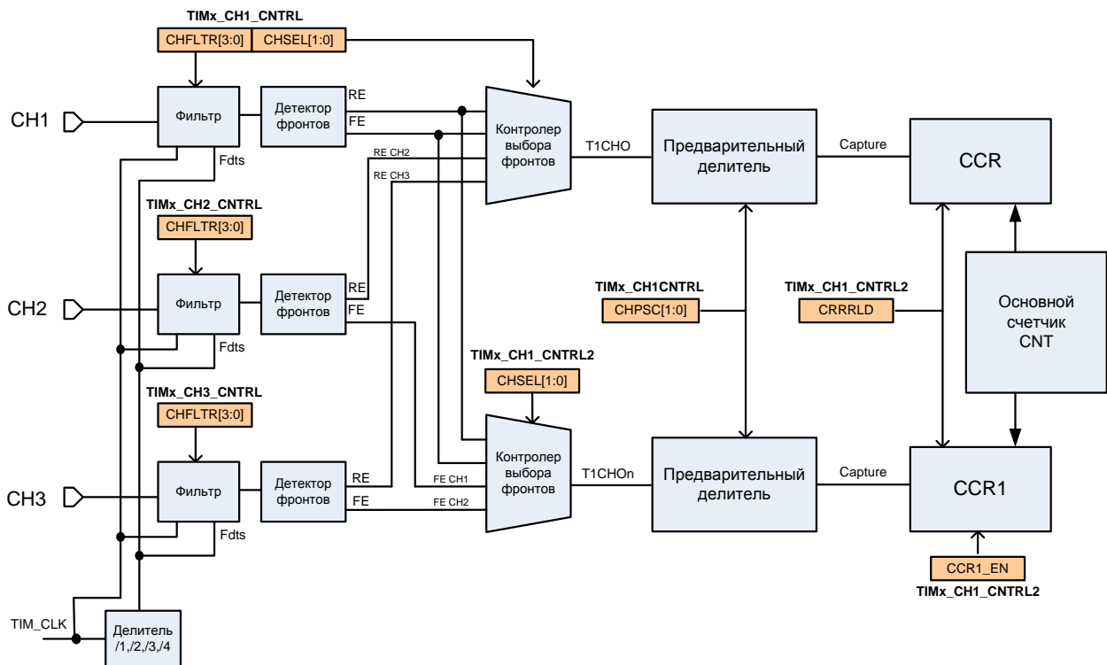
Рисунок 82 – Структурная схема блока захвата на примере канала 1
