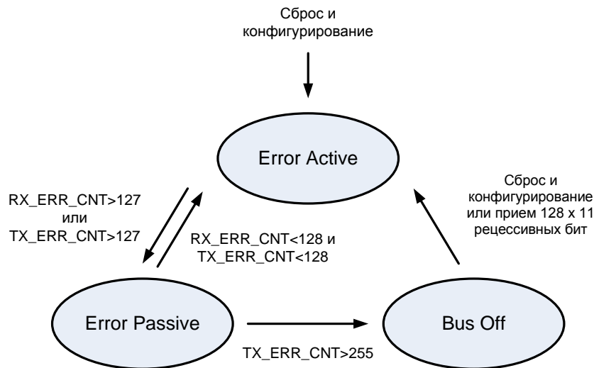
Рисунок 56 – Счетчики ошибок
