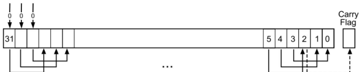
Рисунок 21 – Инструкция LSR # 3
