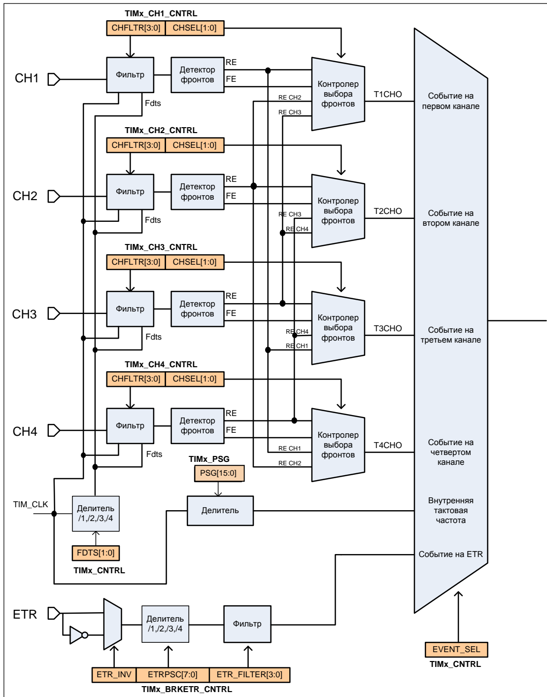
Рисунок 70 – Структурная схема формирования события для счета
