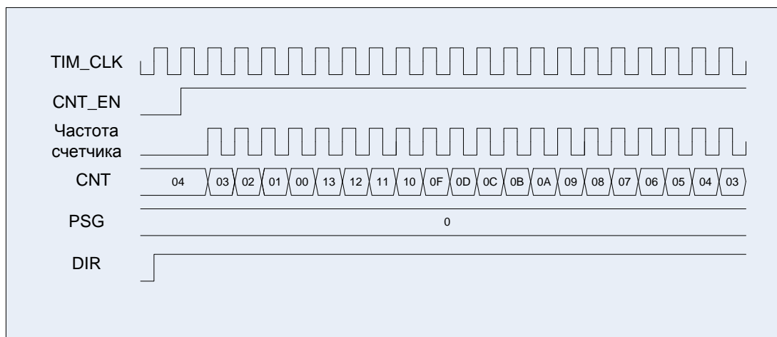
Рисунок 67 – Диаграммы работы таймера, счет вниз от 0x0013 до 0, стартовое значение 0x0004
