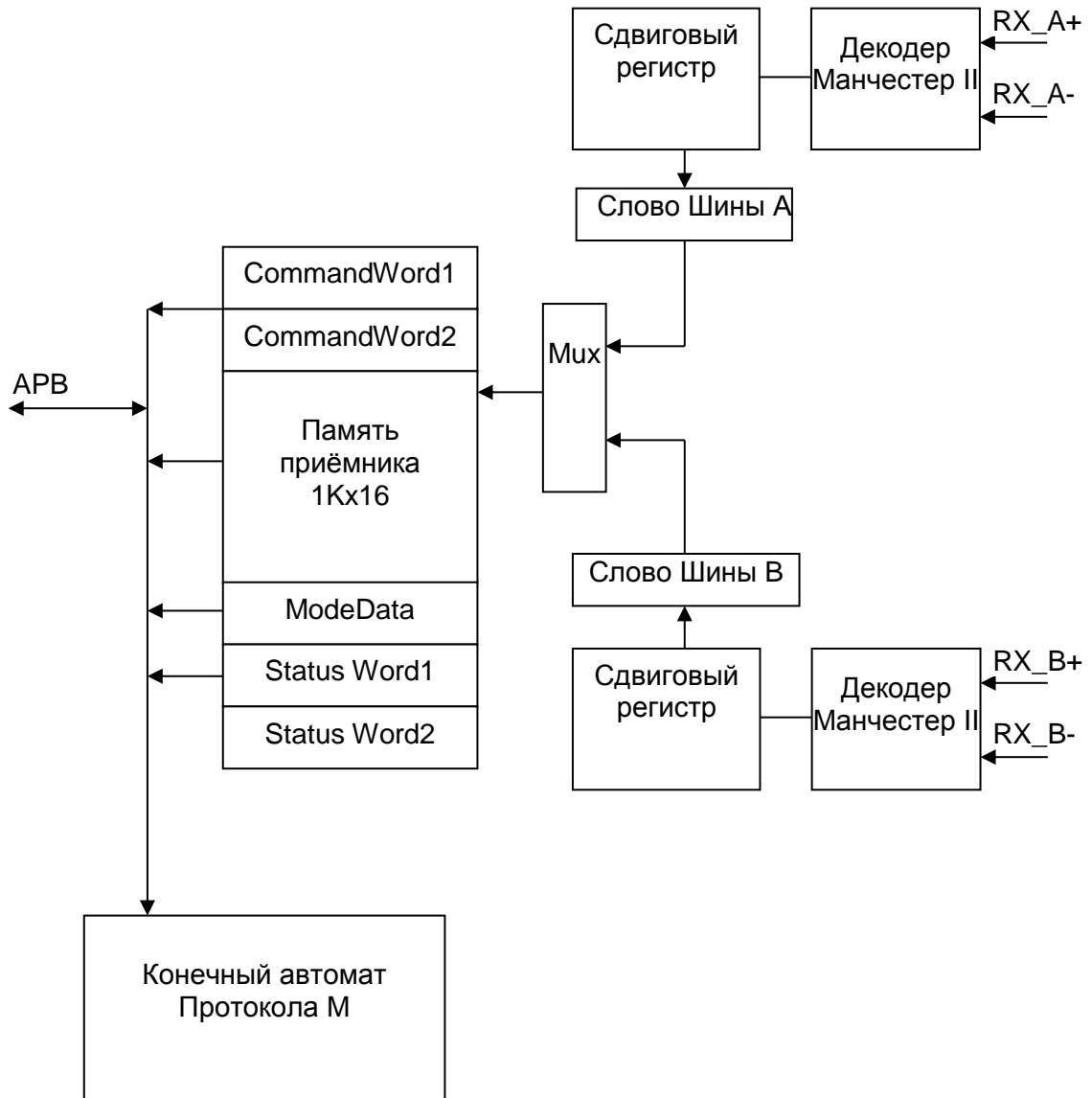
Рисунок 64 – Структурная схема работы в режиме М
