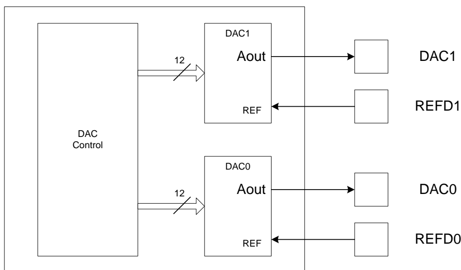
Рисунок 96 – Структурная схема контроллера ЦАП
