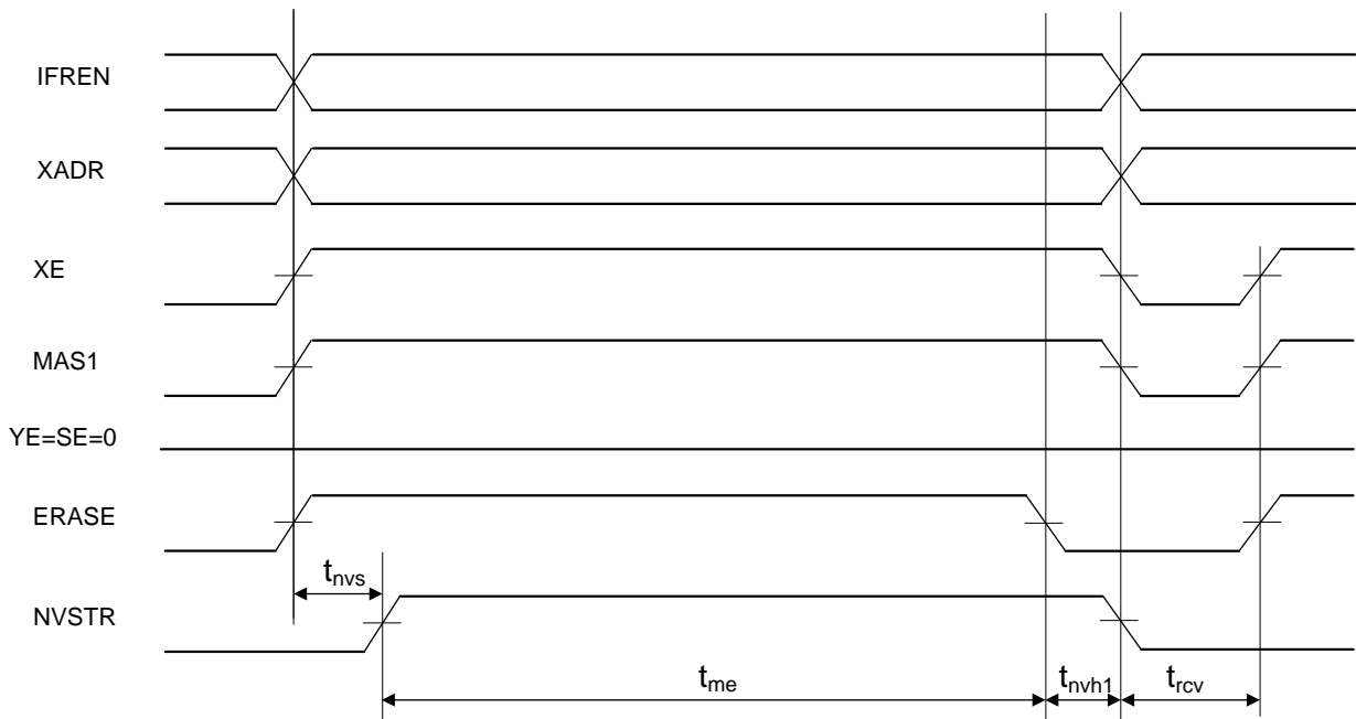
Рисунок 14 – Временная диаграмма стирания памяти
