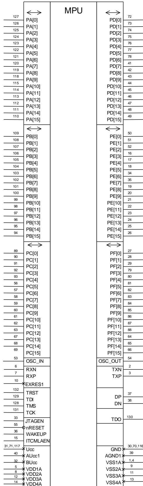
Рисунок 2 – Условное графическое обозначение микросхем в корпусе 4229.132-3
