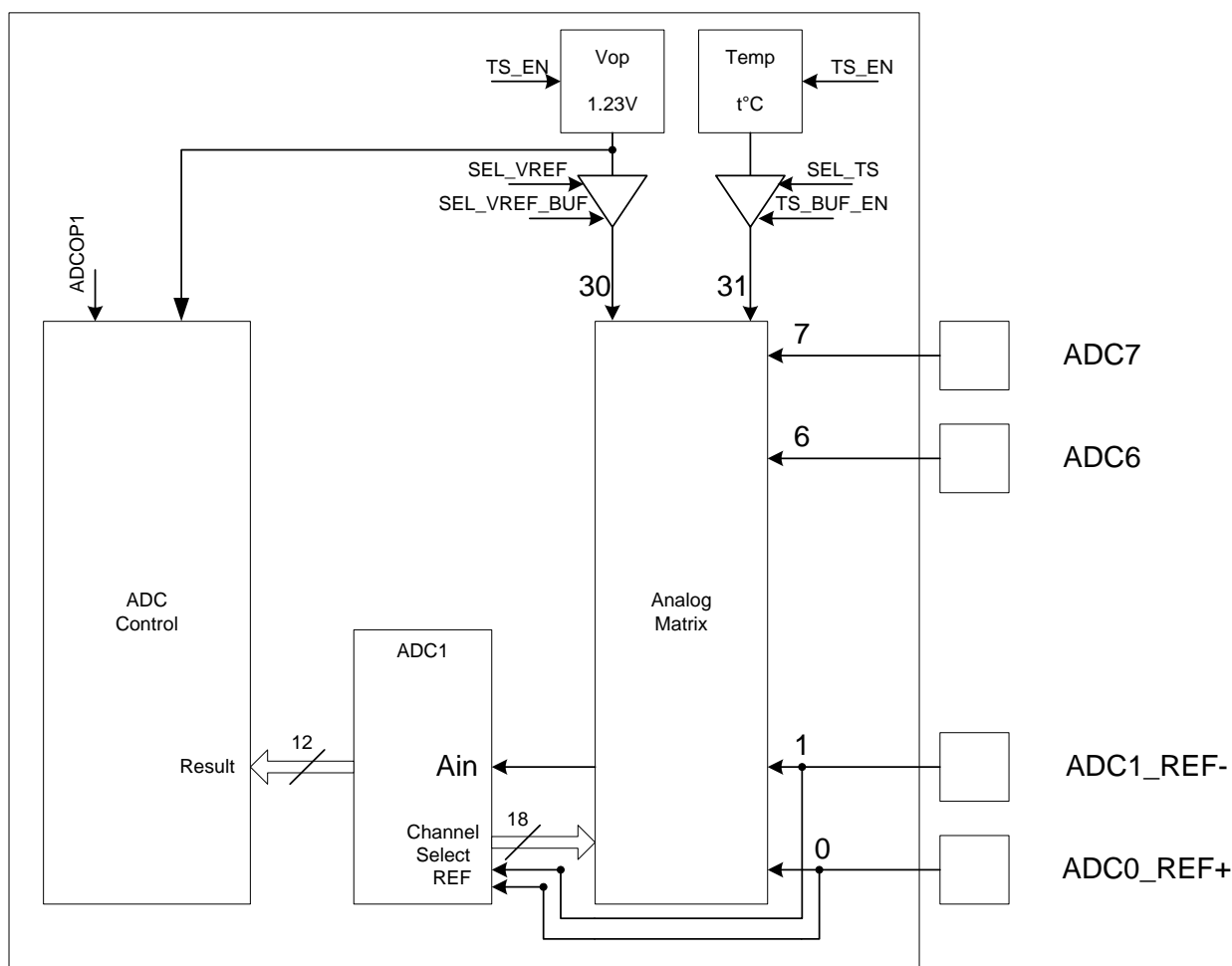
Рисунок 95 – Структурная схема контроллера АЦП
