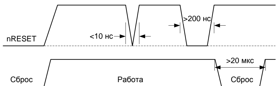
Рисунок 9 – Формирование сигнала сброса
