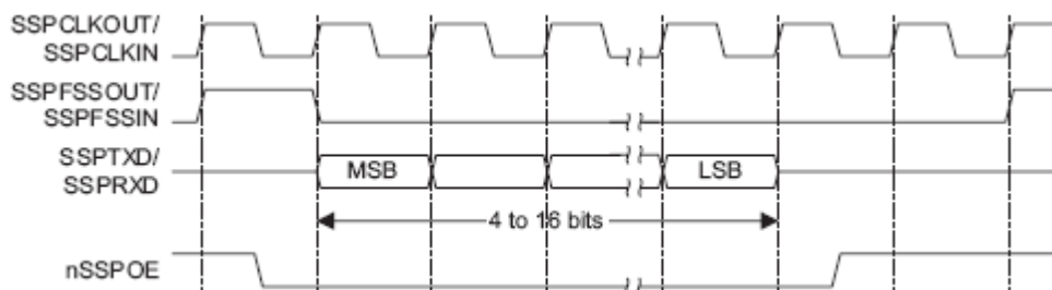
Рисунок 102 – Формат синхронного обмена протокола SSI (единичный обмен)
