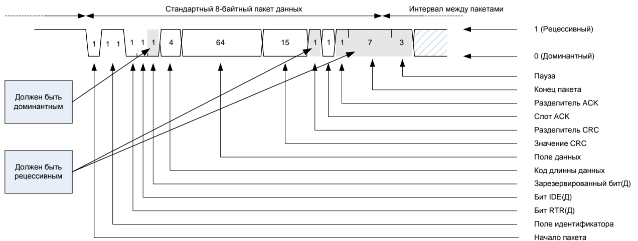
Рисунок 51 – Контроль формата пакета
