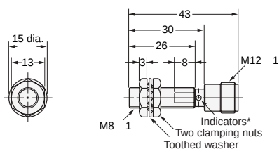
Diagram 18 E2E-X2D□-M1(G) E2E-X1R5E□-M1/E2E-X1R5F□-M1
