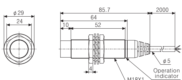
●PRDL18-14D□
