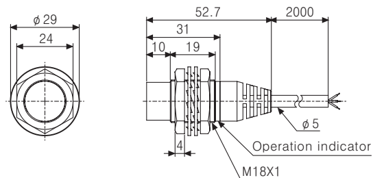
●PRDL18-14D□
