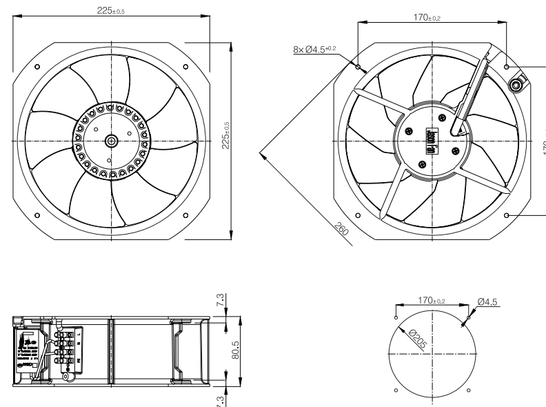
Габаритные и установочные размеры, мм
