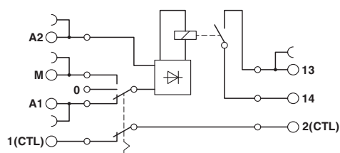
Электрическая схема
