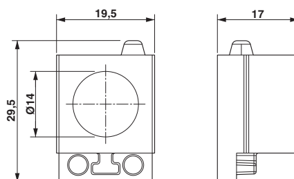
Чертеж
