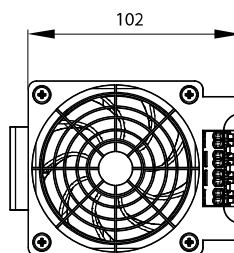
Габаритные и установочные размеры, мм
