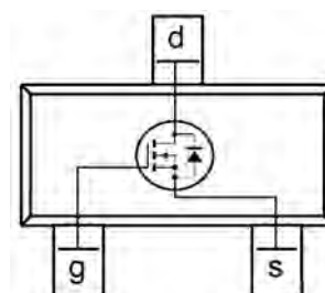
SOT-23
