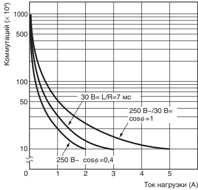
Кривая испытания на срок службы (справочные значения)
